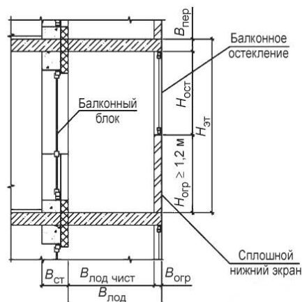
Принципиальная схема компоновки лоджии (вариант со сплошным нижним экраном)
