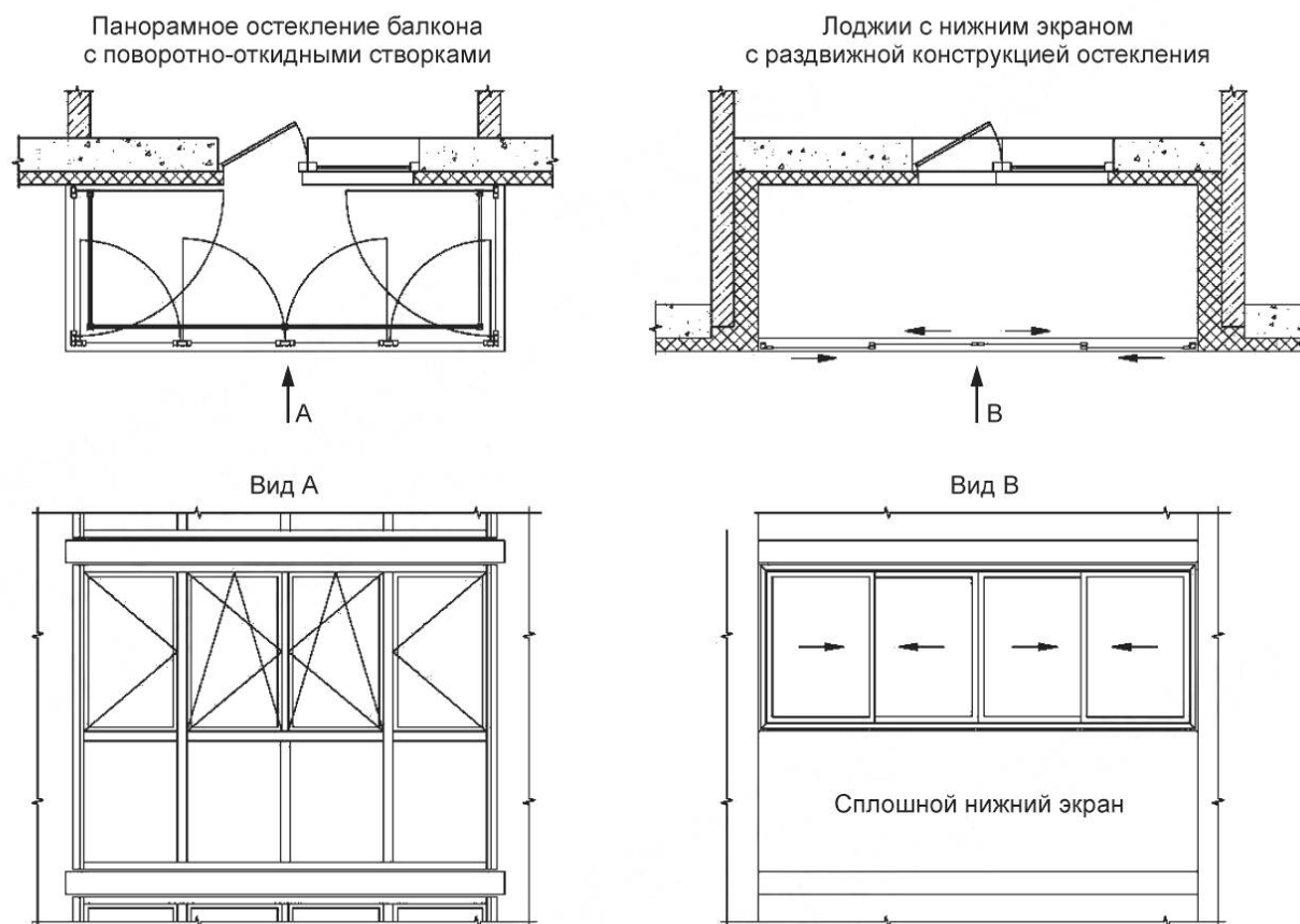
Рисунок Д.2 — Примеры конструкций наружного остекления
