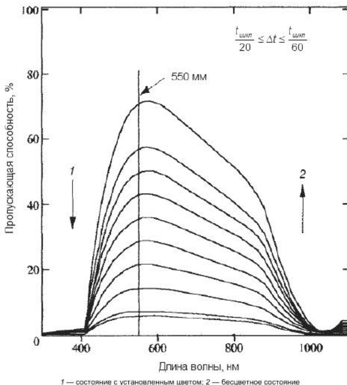
Рисунок 4 — Спектры пропускания в течение набора цвета и снятия цвета в интервале от t_{\text{ц/лп}}/20 до t_{\text{ц/лп}}/60
