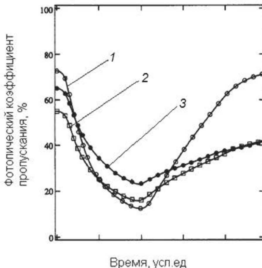
Рисунок 5 — График зависимости фотопической пропускной способности от времени
