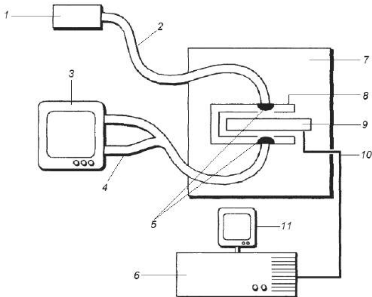
1 — лампа накаливания (с вольфрамовой нитью); 2 — оптоволоконный кабель; 3 — спектрофотометр с фотодиодной матрицей, подключенный к компьютеру; 4 — кабель-разветвитель оптоволоконный; 5 — коллимирующая линза; 6 — многоканальная цифровая автоматизированная система управления и сбора данных; 7 — термощаф; 8 — держатель образца; 9 — стекло с ЭХП; 10 — электрические выводы и кабели термопар; 11 — компьютер
