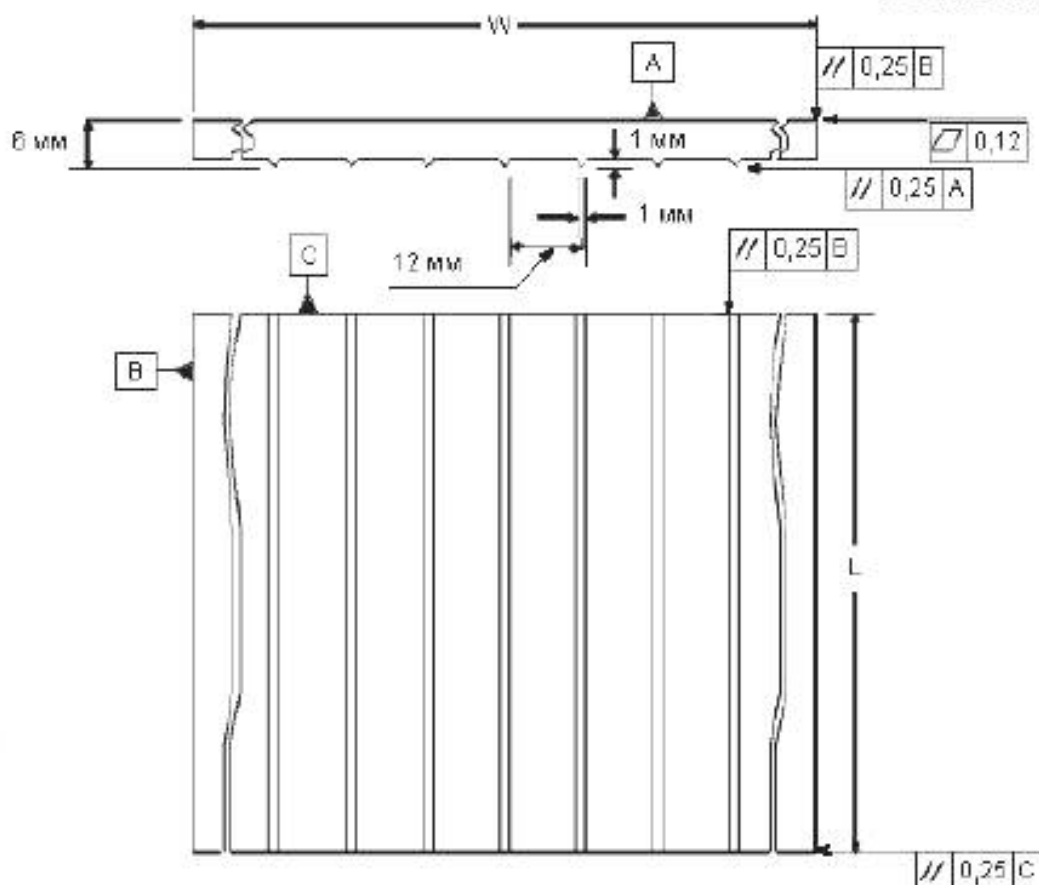
L — длина пластины; W — ширина пластины Рисунок 1 — Зубчатая пластина
