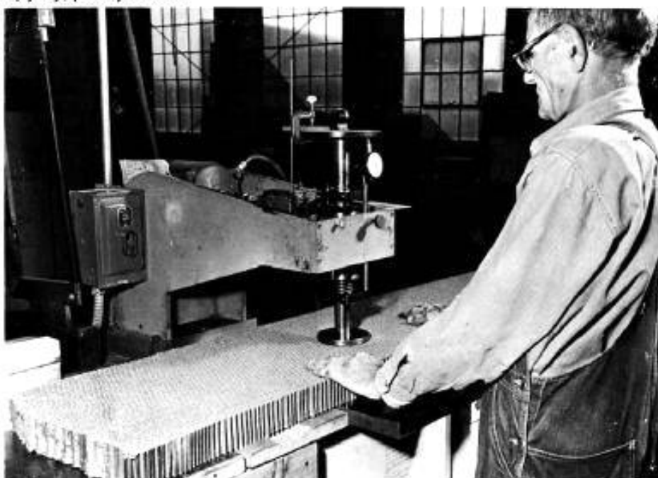
Рисунок 2 — Толщиномер дискового типа
