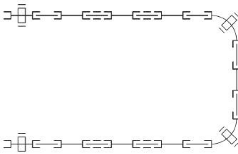
в) Альтернативная схема сборки образца для напорных труб d_s \geq 63 мм
