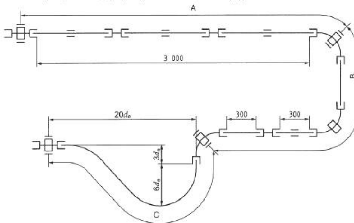
а) Схема сборки образца
