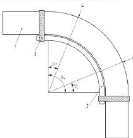
1 – изолированная труба; 2 – шаблон; 3 – зажимы; 4 – позиции измерения овальности
