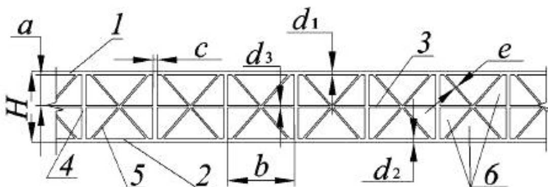
1 — внешний лицевой слой; 2 — внешний нелицевой слой; 3 — внутренний горизонтальный слой; 4 — вертикальные ребра жесткости; 5 — наклонные ребра жесткости; 6 — каналы; H — толщина панели; a — расстояние между горизонтальными слоями; b — расстояние между вертикальными ребрами жесткости; d_1 — толщина внешнего лицевого слоя; d_2 — толщина внешнего нелицевого слоя; d_3, d_4 \dots d_n — толщина внутренних горизонтальных слоев; c — толщина вертикальных ребер жесткости; e — толщина наклонных ребер жесткости
