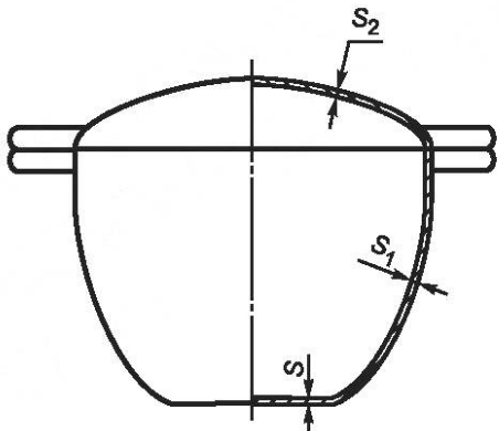
Рисунок 8 — Казан
