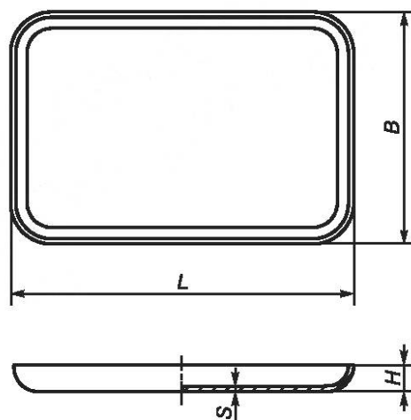
Рисунок 9 — Противень
