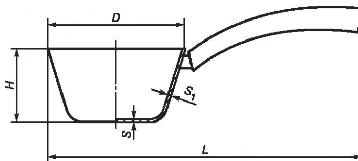
Рисунок 7 — Ковш
