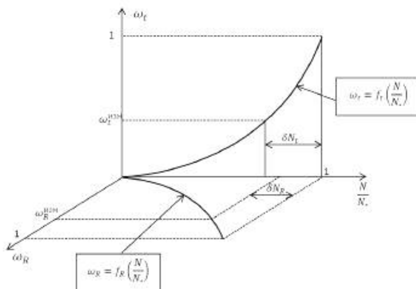
Рисунок 1 — Определение относительного остаточного ресурса
