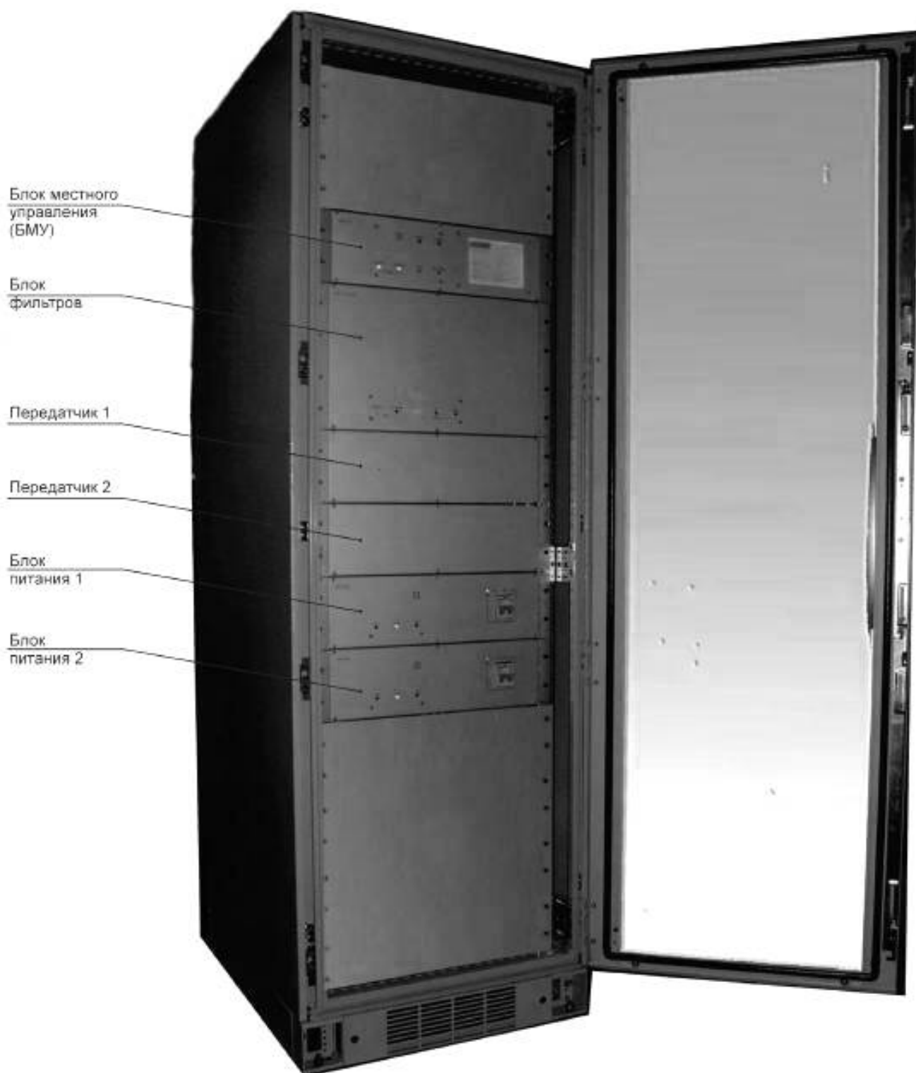
Рисунок 1 — Общий вид радиомаяка «Янтарь-1000»
