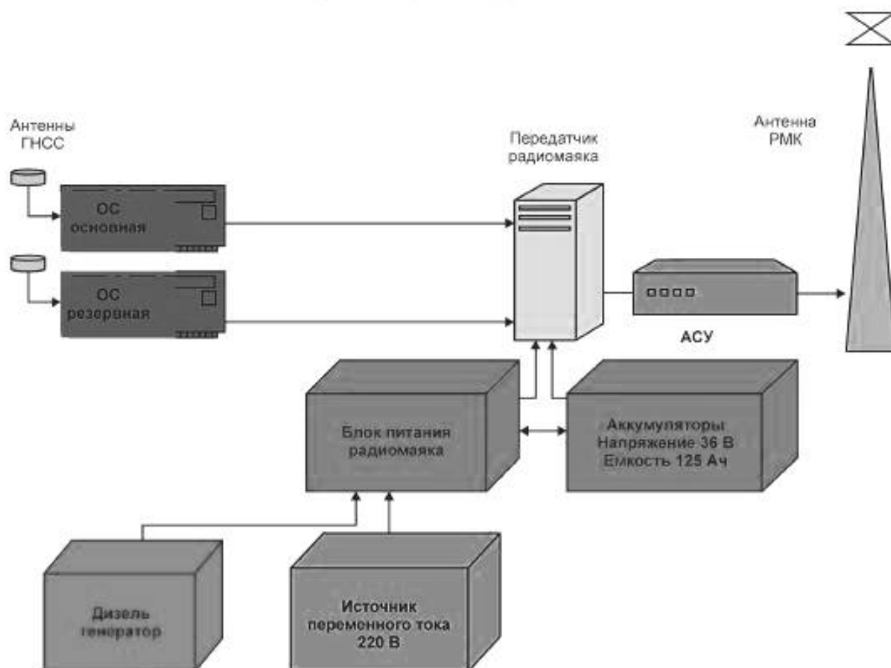
Рисунок 3 — Схема межблочных соединений и питания радиомаяка
