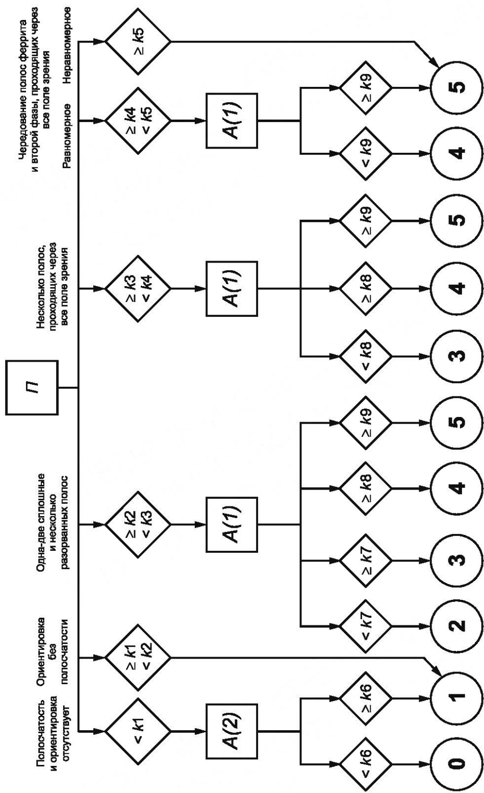
Рисунок Г.2 — Дерево решений для назначения балла полосчатости структуры Таблица Г.1 — Предельные значения коэффициентов полосчатости, анизотропии феррита и анизотропии «второй фазы»
