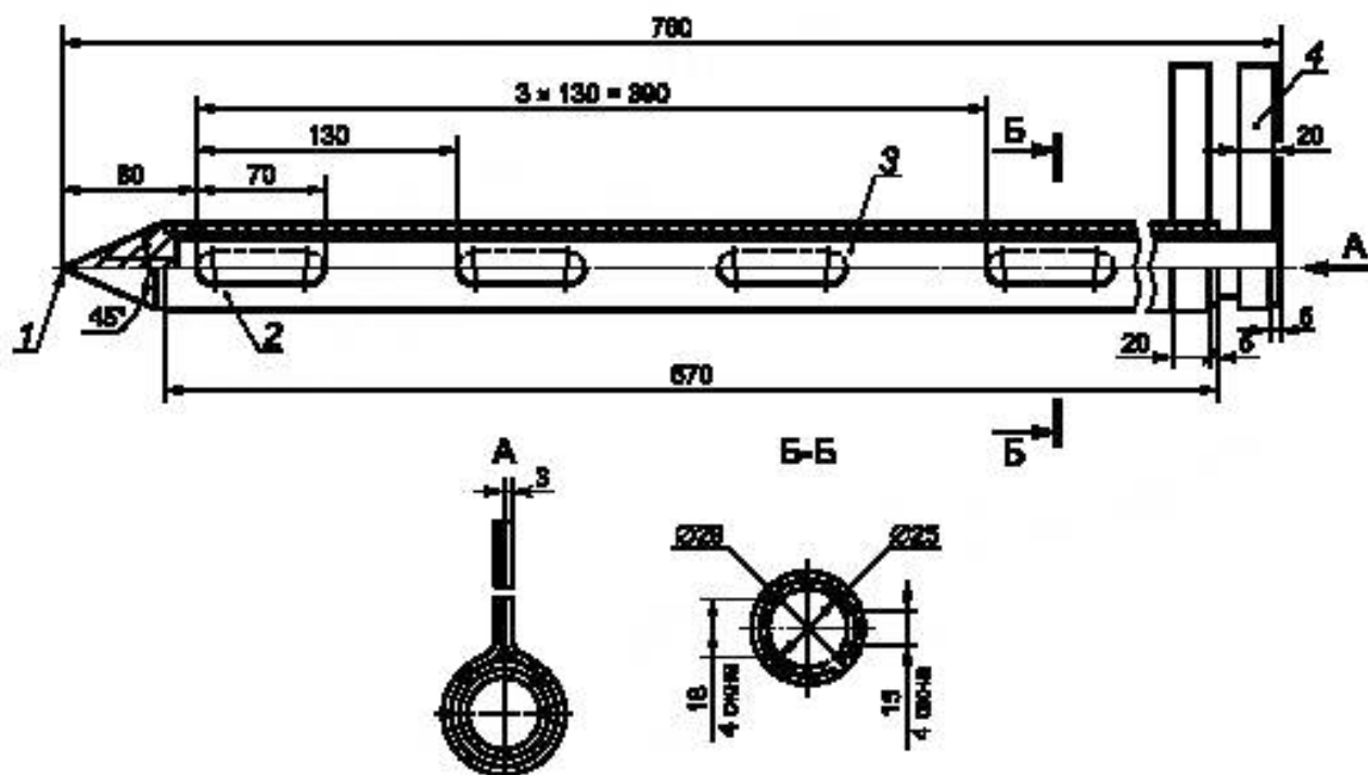
1 — наконечник; 2 — наружная труба; 3 — внутренняя труба; 4 — ручка
