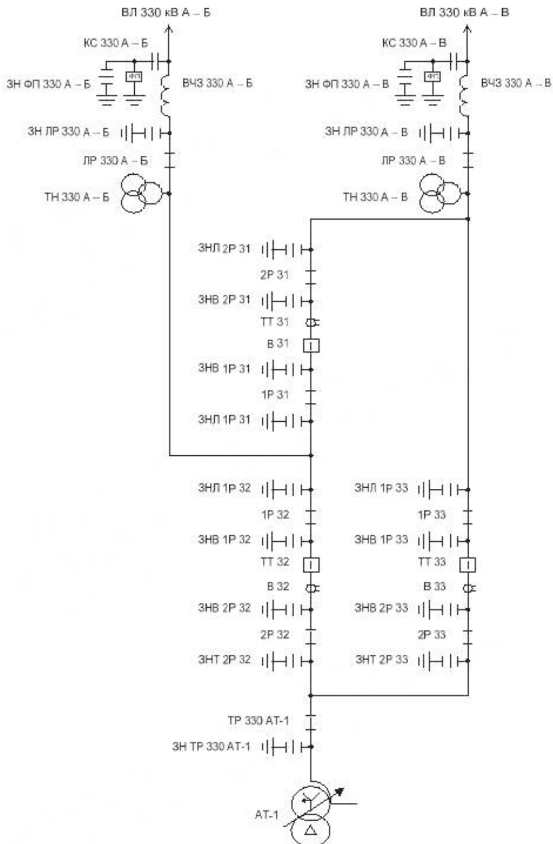
Рисунок Б.3 – Схема РУ 330 кВ типа «треугольник»
