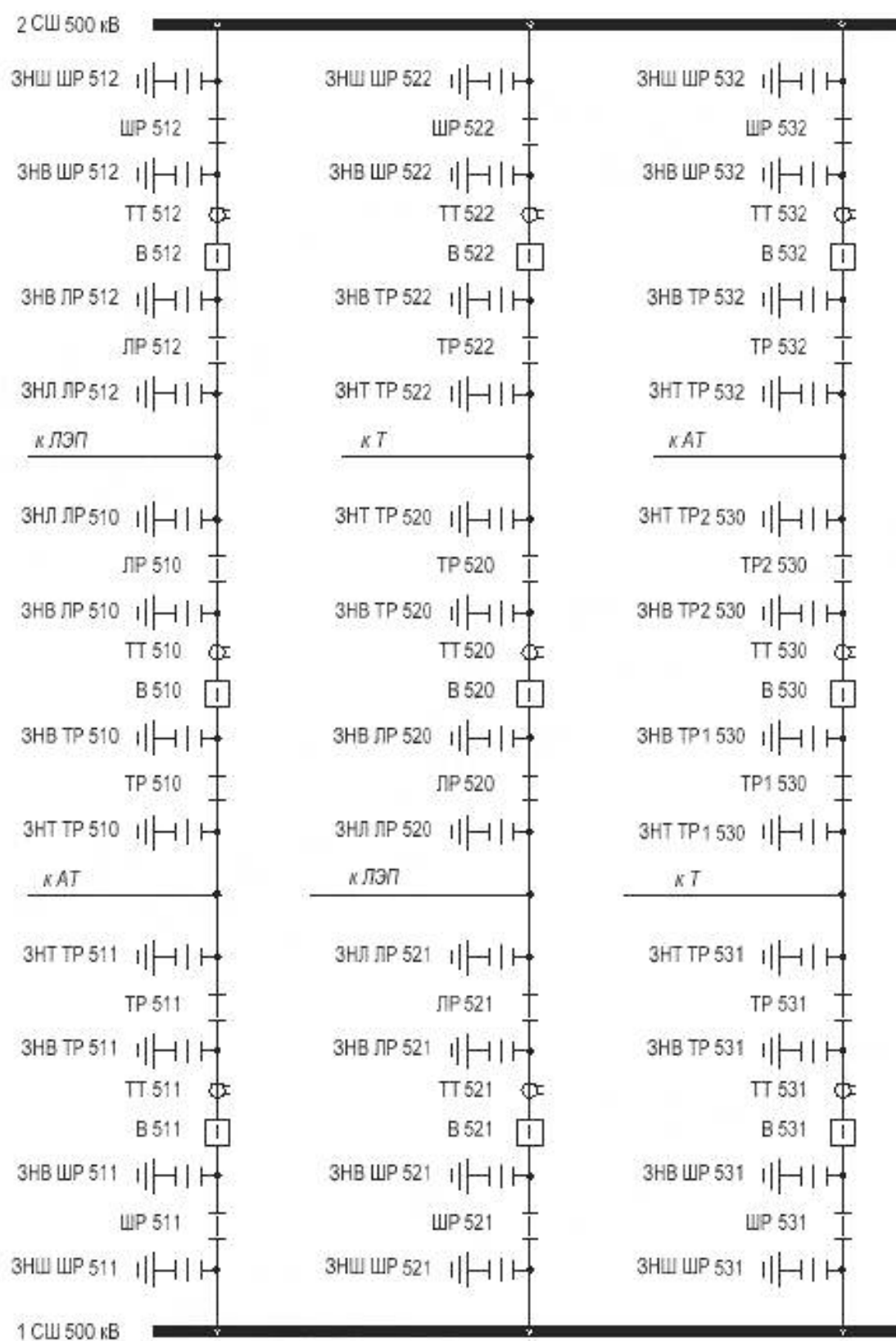
Рисунок Б.4 – Схема РУ 500 кВ типа «трансформаторы – шины с полуторным присоединением линий»
