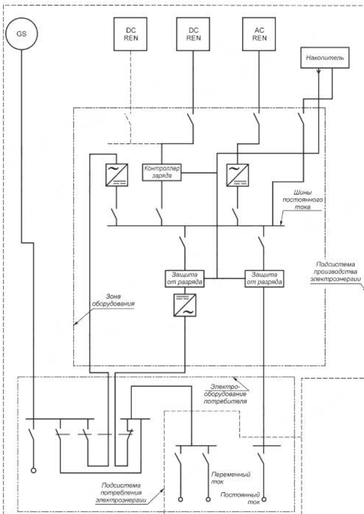
Рисунок Д.8 — Система типа T 4 I
