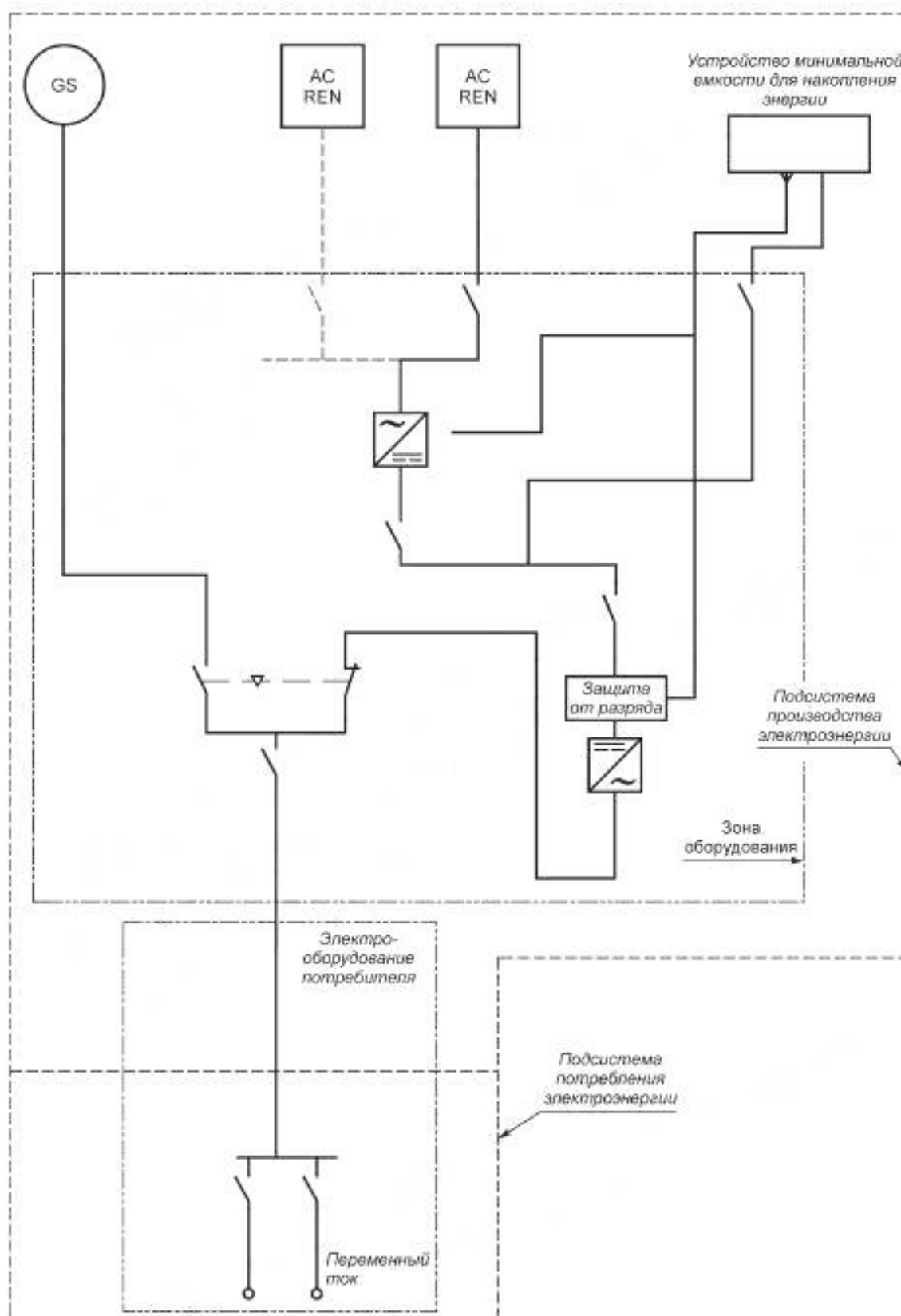
Рисунок Д.7 — Система типа T 3 -b
