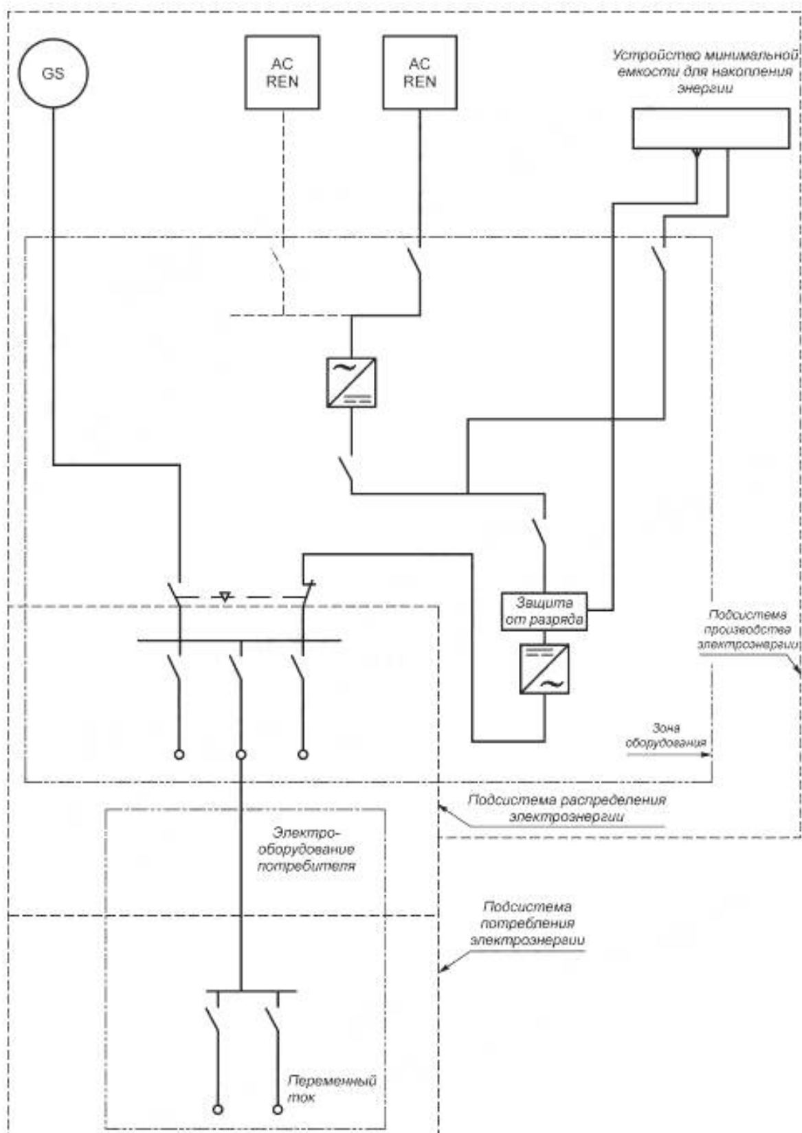
Рисунок Д.14 — Система типа T 3 C-b
