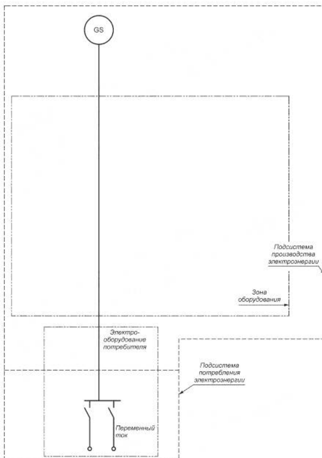
Рисунок Д.9 — Система типа T 5 I
