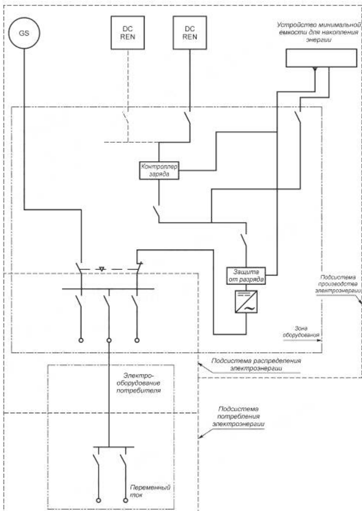
Рисунок Д.13 — Система типа Т 3 С-а
