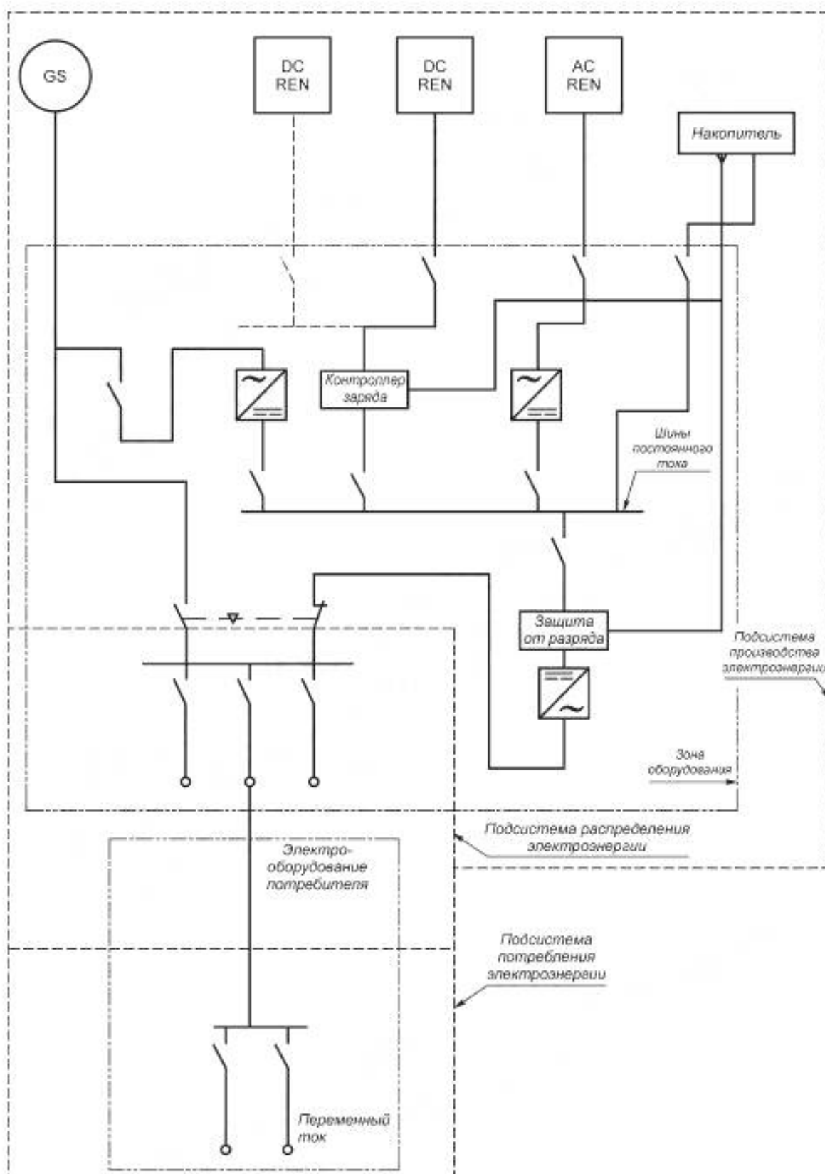
Рисунок Д.15 — Система типа T 4 C-a
