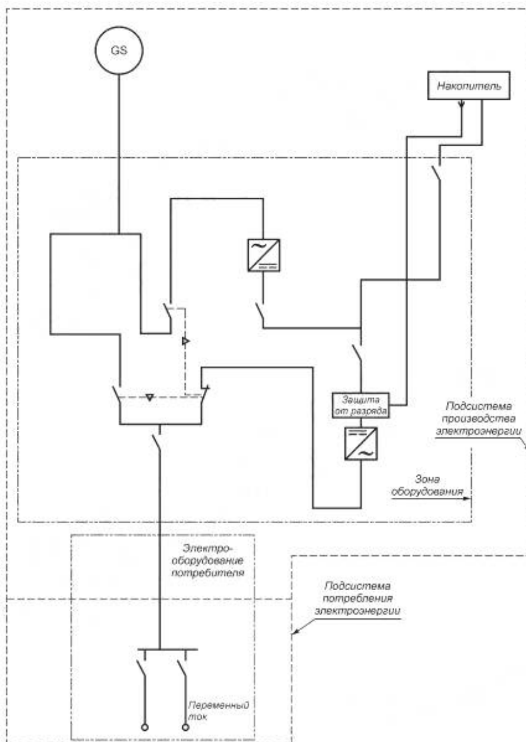
Рисунок Д.10 — Система типа T 6I
