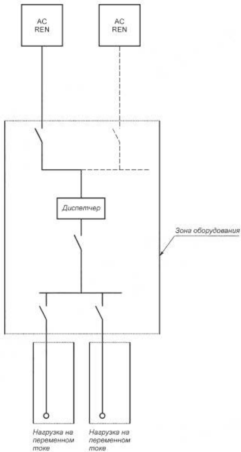
Рисунок Д.2 — Система типа T 1 -b
