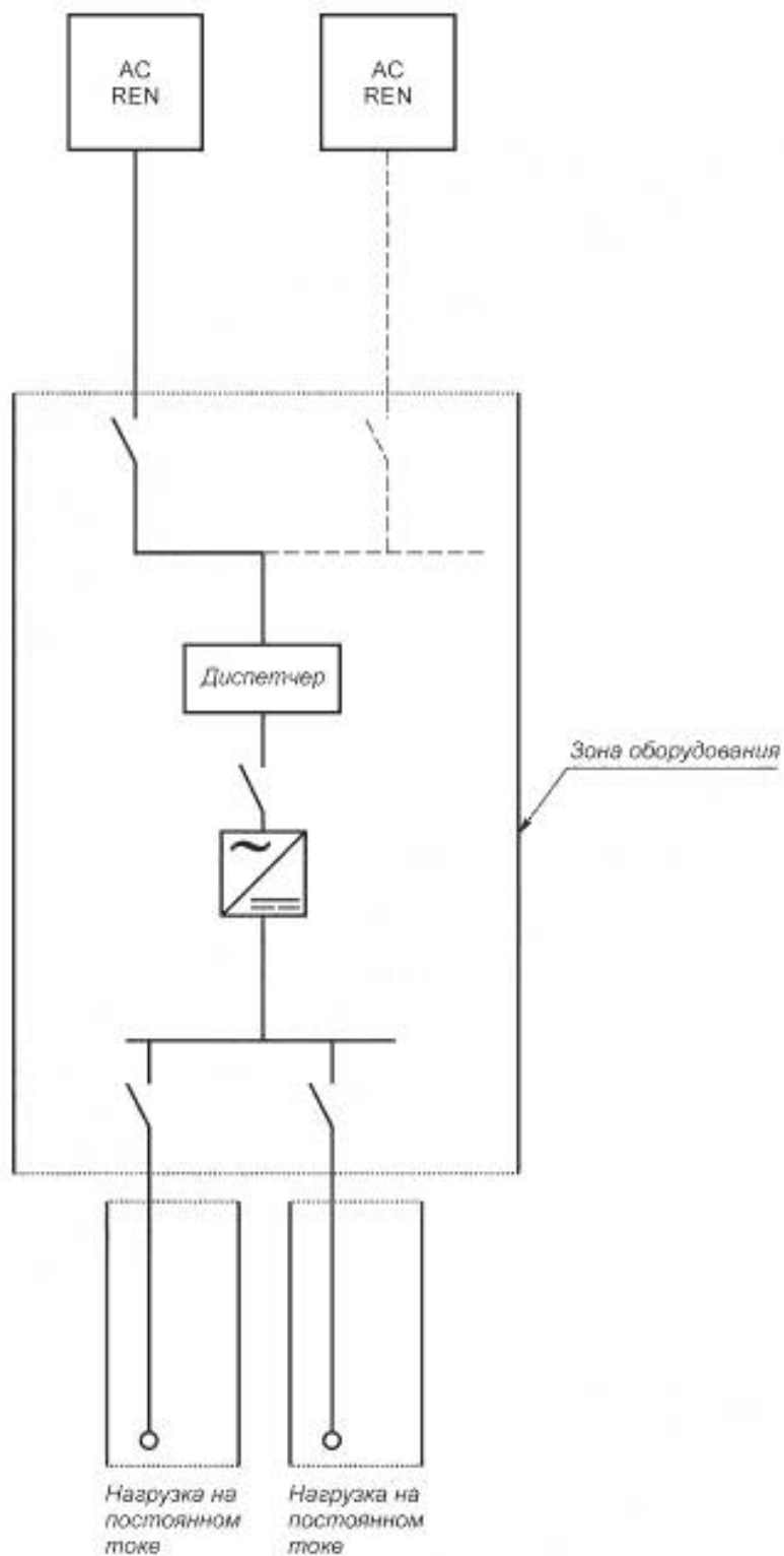
Рисунок Д.3 — Система типа T 1 -с
