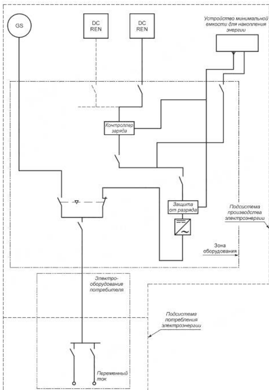
Рисунок Д.6 — Система типа T 3I -а
