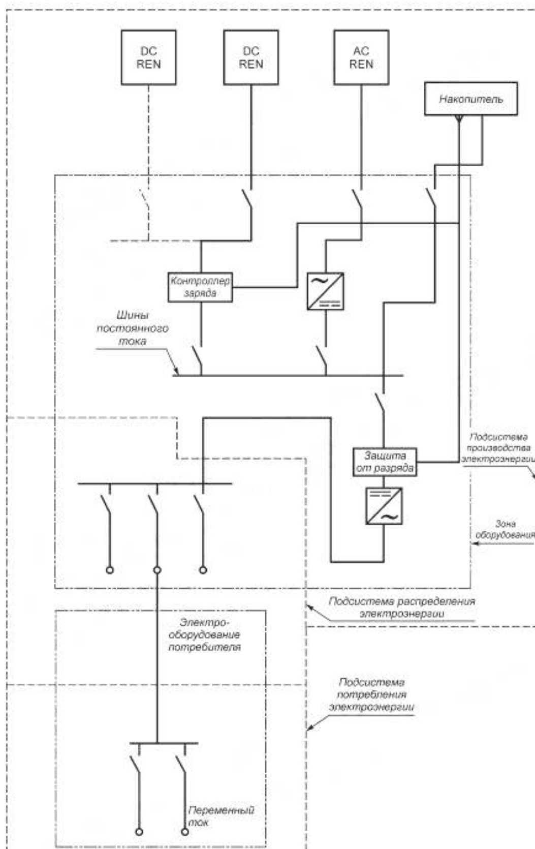
Рисунок Д.12 — Система типа T 2 C
