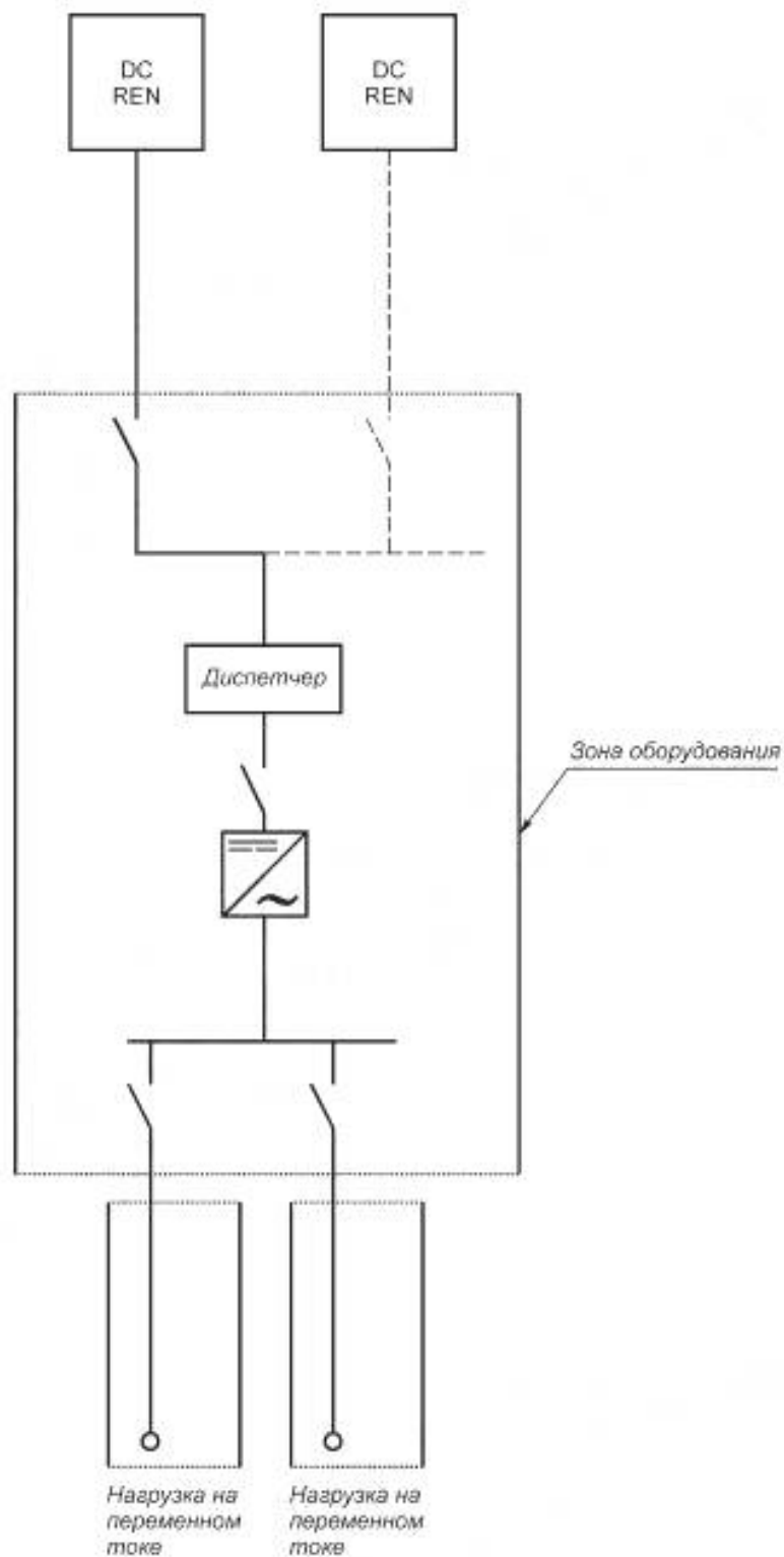
Рисунок Д.4 — Система типа T 1 I-d.
