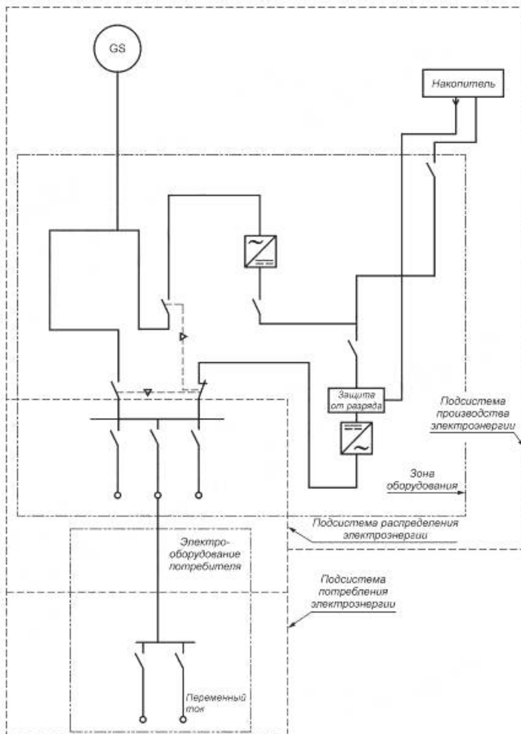
Рисунок Д.18 — Система типа T 6 C
