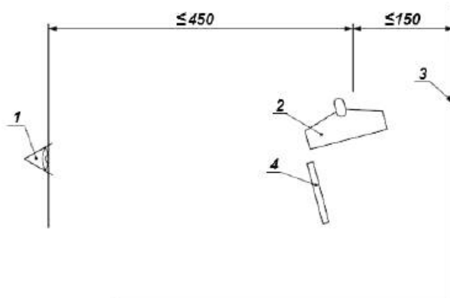
Рисунок 1 – Проверка отражения
