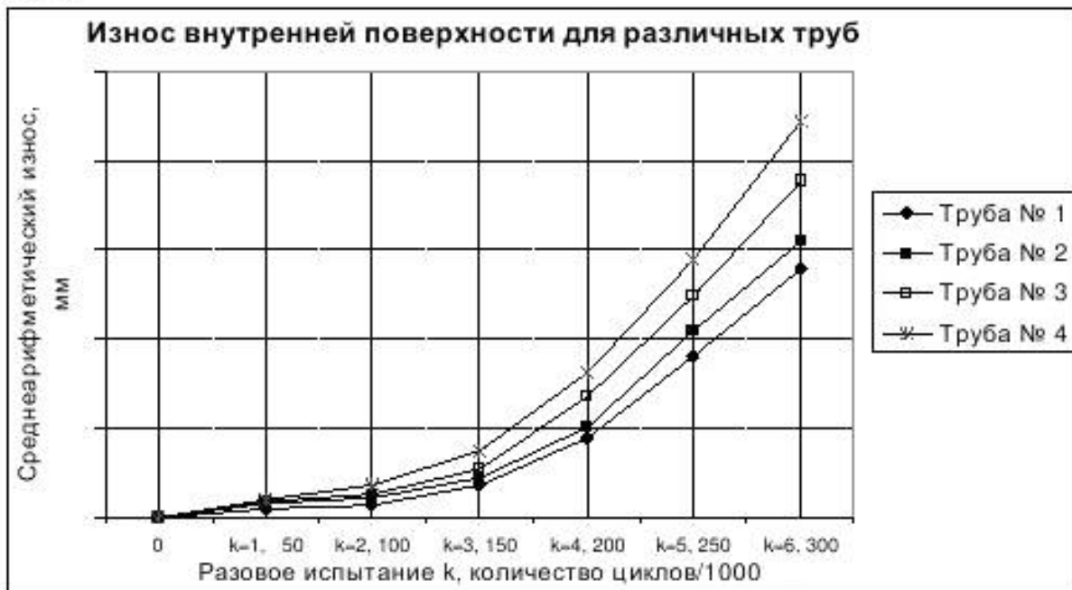
Рисунок 4 – Зависимость износа от количества испытательных циклов
