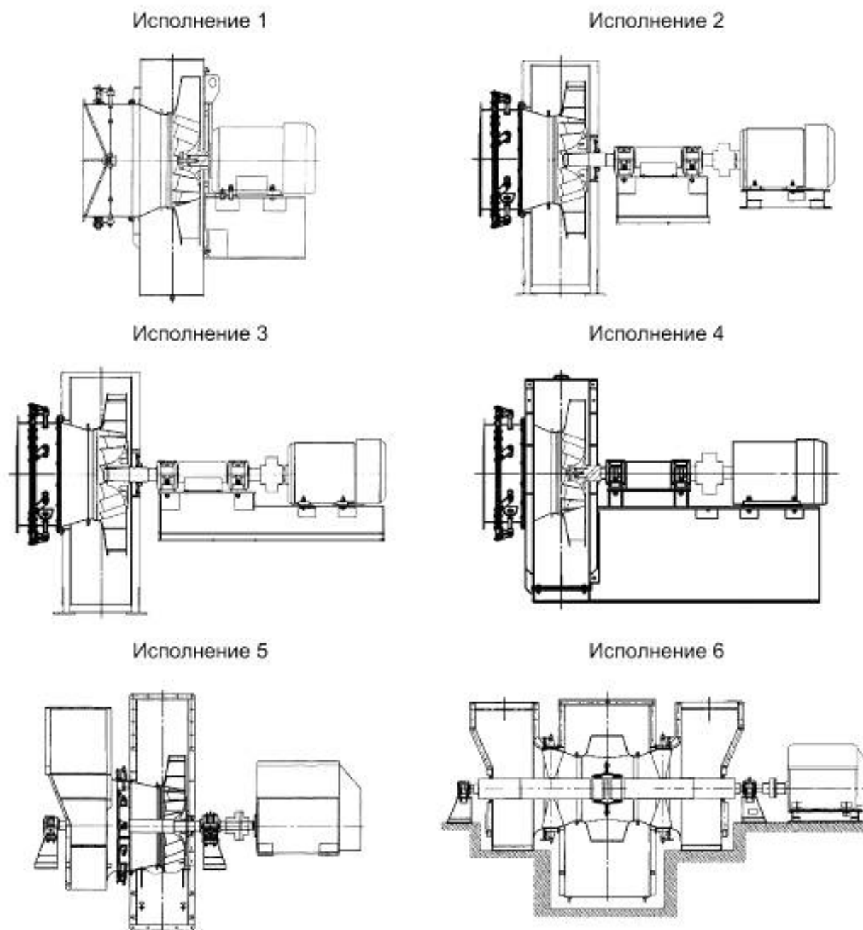
Рисунок 1 — Конструктивные исполнения центробежных ТДМ
