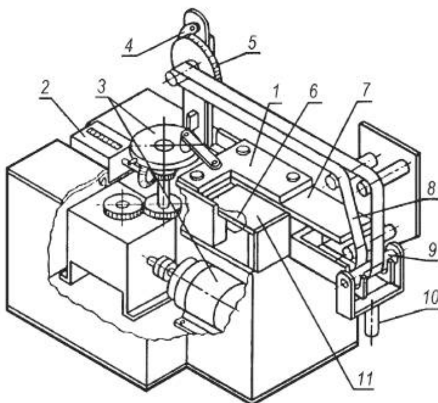
Рисунок 2 – Прибор типа ИК – 1
