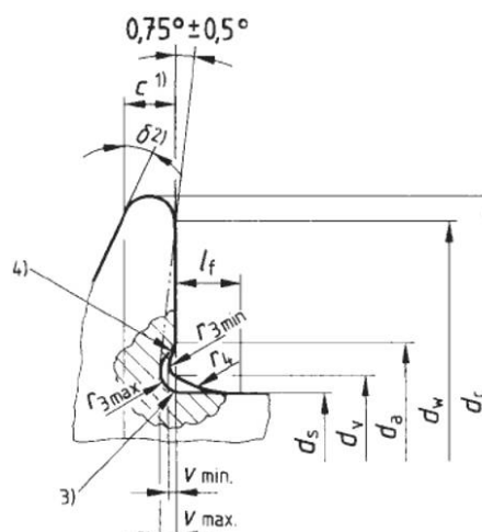
Тип U с поднутрением (по запросу или дополнительный)
