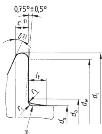
Рисунок 2 - Болт с шестигранной головкой с фланцем – уменьшенный стержень, тип R (по запросу)
