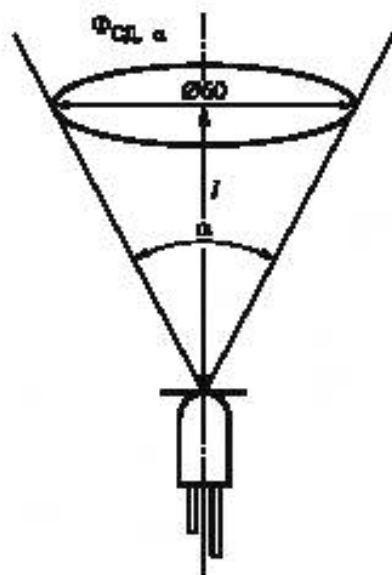
Рисунок 2 — Схема для измерения частичного светового потока
