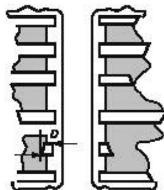
D — поясок площадки внутреннего слоя
