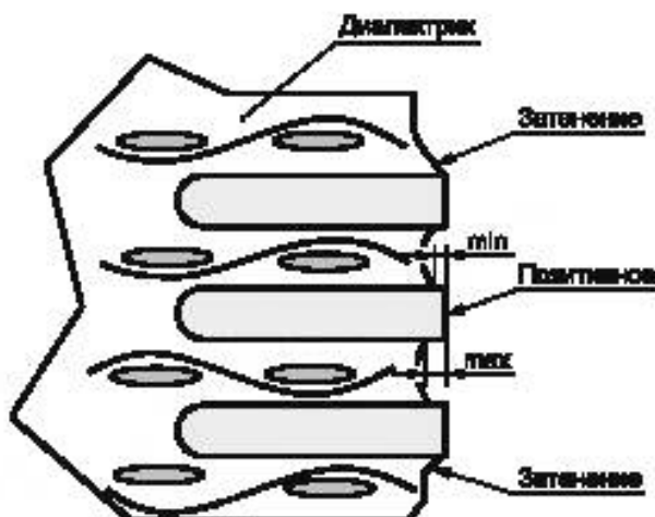
Рисунок 8 — Измерение значения травления диэлектрика
