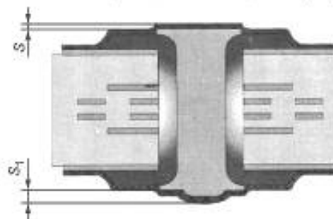
Рисунок 13 — Измерение толщины выступов «крышки»
