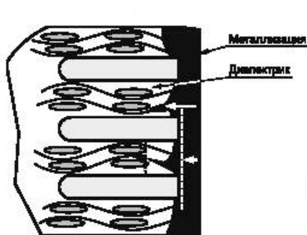
Рисунок 7 — Травление диэлектрика
