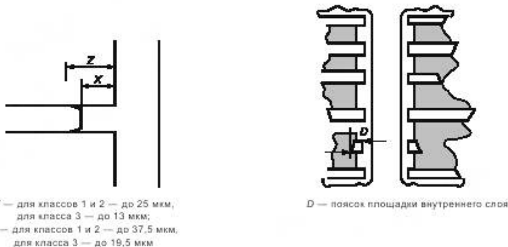
Рисунок 9 — Измерение значения негативного подтравливания
