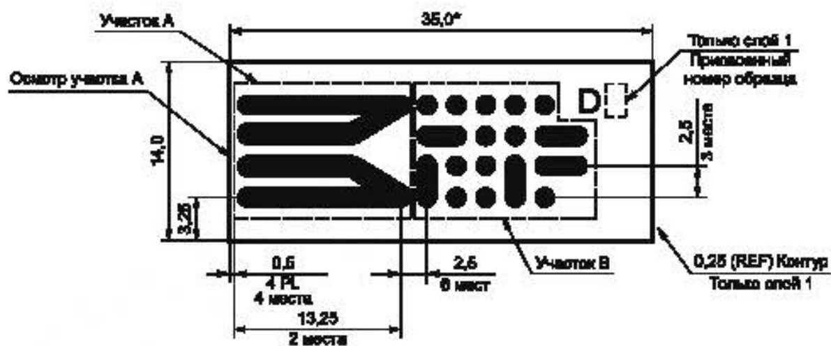
Рисунок В.4 — Тест-кулон D
