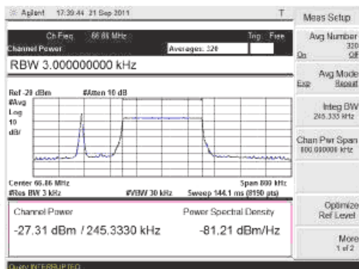
Рисунок В.11 – Сигнал для измерения мощности
