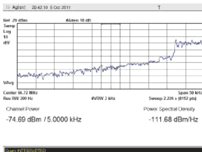
Рисунок В.25 – Плотность мощности минус 111,7 дБм/Гц на частоте f_{(10-140)}
