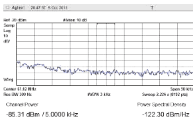
Рисунок В.32 – Плотность мощности минус 120,6 дБм/Гц на частоте f_{(10+155)}
