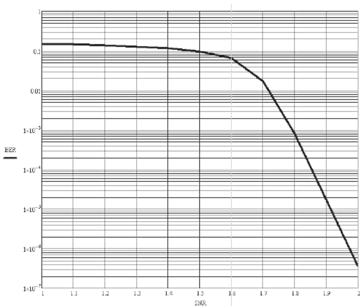
Рисунок Б.1 – График зависимости BER от ОСШ
