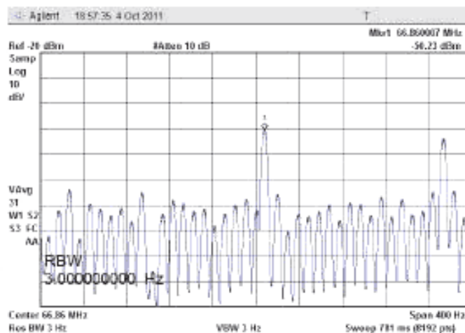
Рисунок В.38 – Полоса сканирования (Span) 400 Гц
