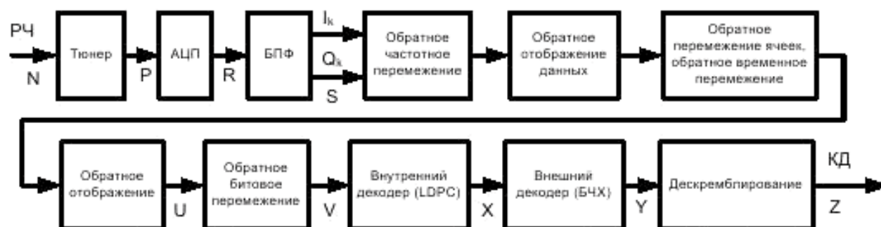
Рисунок 2 – Функциональная схема приемной части системы RABIS (приемник)
