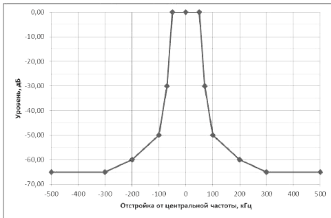
Рисунок А.1 – Маска огибающей внеполосных радиоколечаний для условной ширины полосы частот 100 кГц
