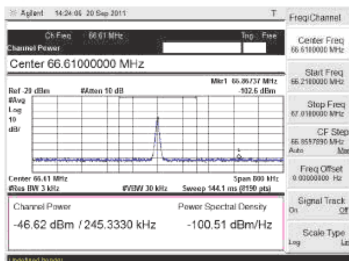
Рисунок В.13 – Измерение мощности синусоидального сигнала
