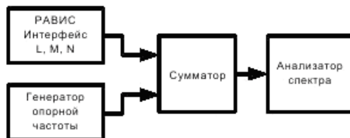
Рисунок 3 – Схема измерения точности настройки по РЧ
