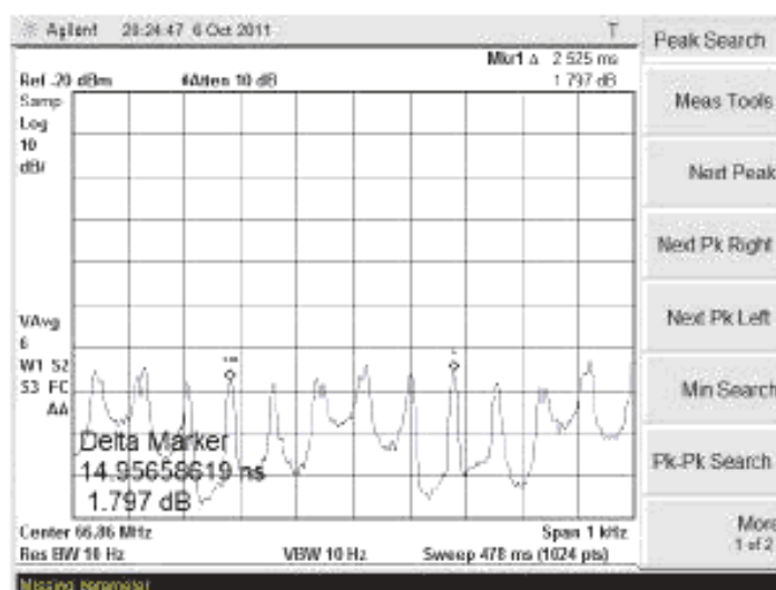
Рисунок В.8 – Спектр ИС «РПН» в полосе сканирования (Span) 1 кГц
