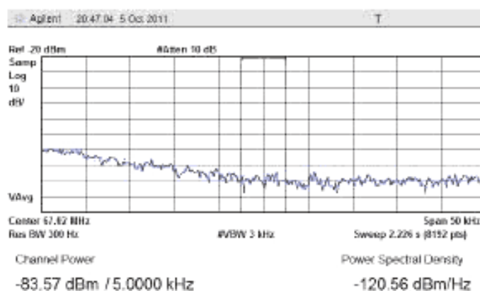
Рисунок В.31 – Плотность мощности минус 121,1 дБм/Гц на частоте f_{(10+150)}
