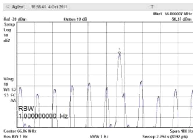
Рисунок В.39 – Полоса сканирования (Span) 100 Гц
