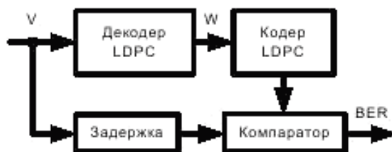
Рисунок 6 – Измерение BER до канального декодера LDPC
