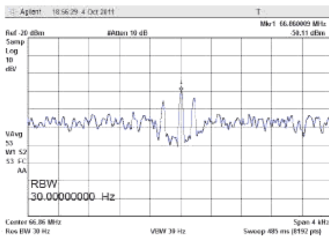
Рисунок В.37 – Полоса сканирования (Span) 4 кГц
