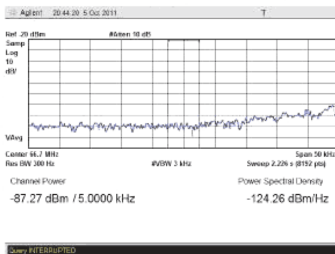
Рисунок В.21 – Плотность мощности минус 124,3 дБм/Гц на частоте f_{(10-150)}
