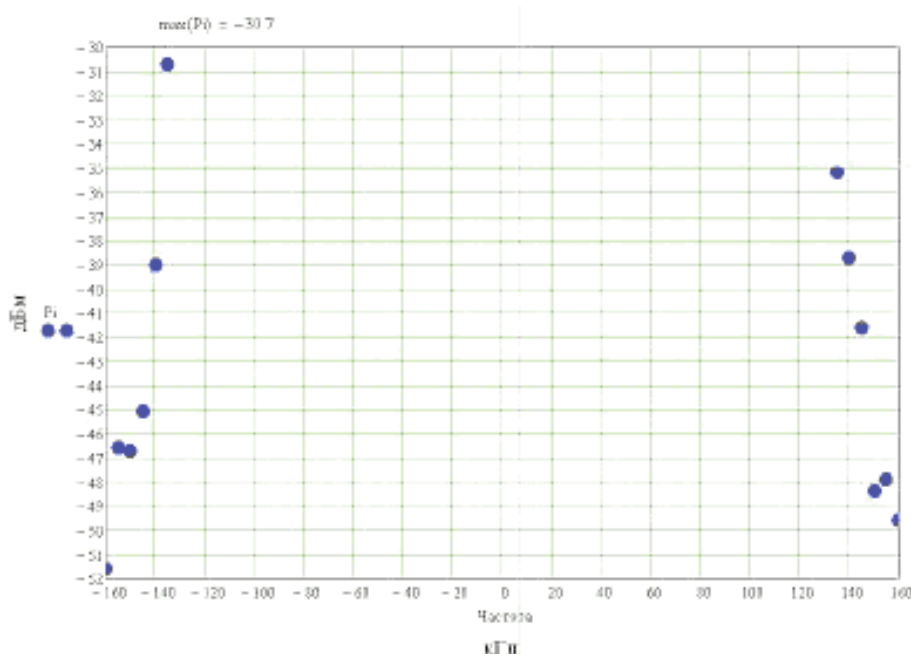
Рисунок В.34 – Разности спектральных плотностей мощности
