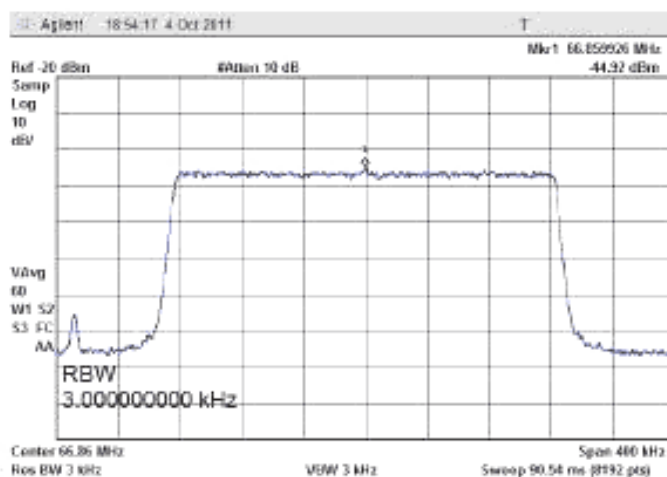
Рисунок В.35 – Полоса сканирования (Span) 400 кГц
