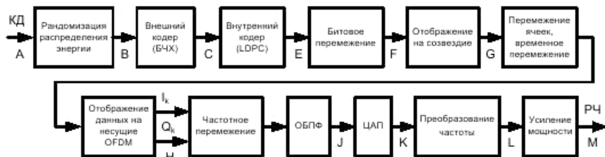
Рисунок 1 – Функциональная схема передающей части системы РАВИС (передатчик)
