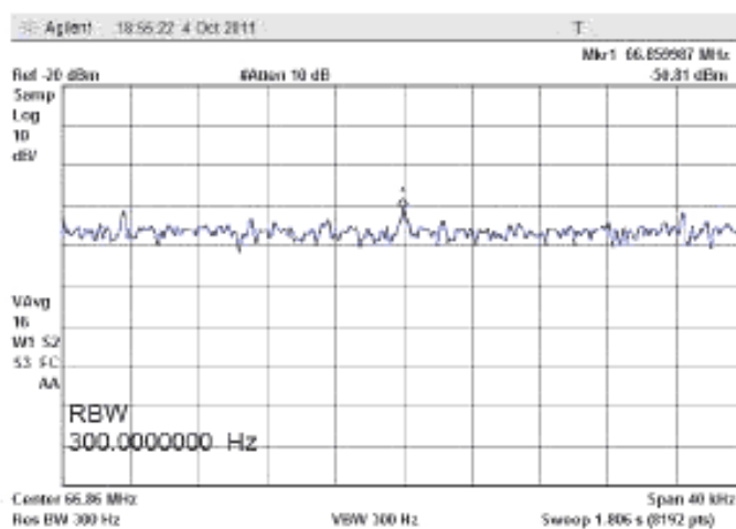
Рисунок В.36 – Полоса сканирования (Span) 40 кГц
