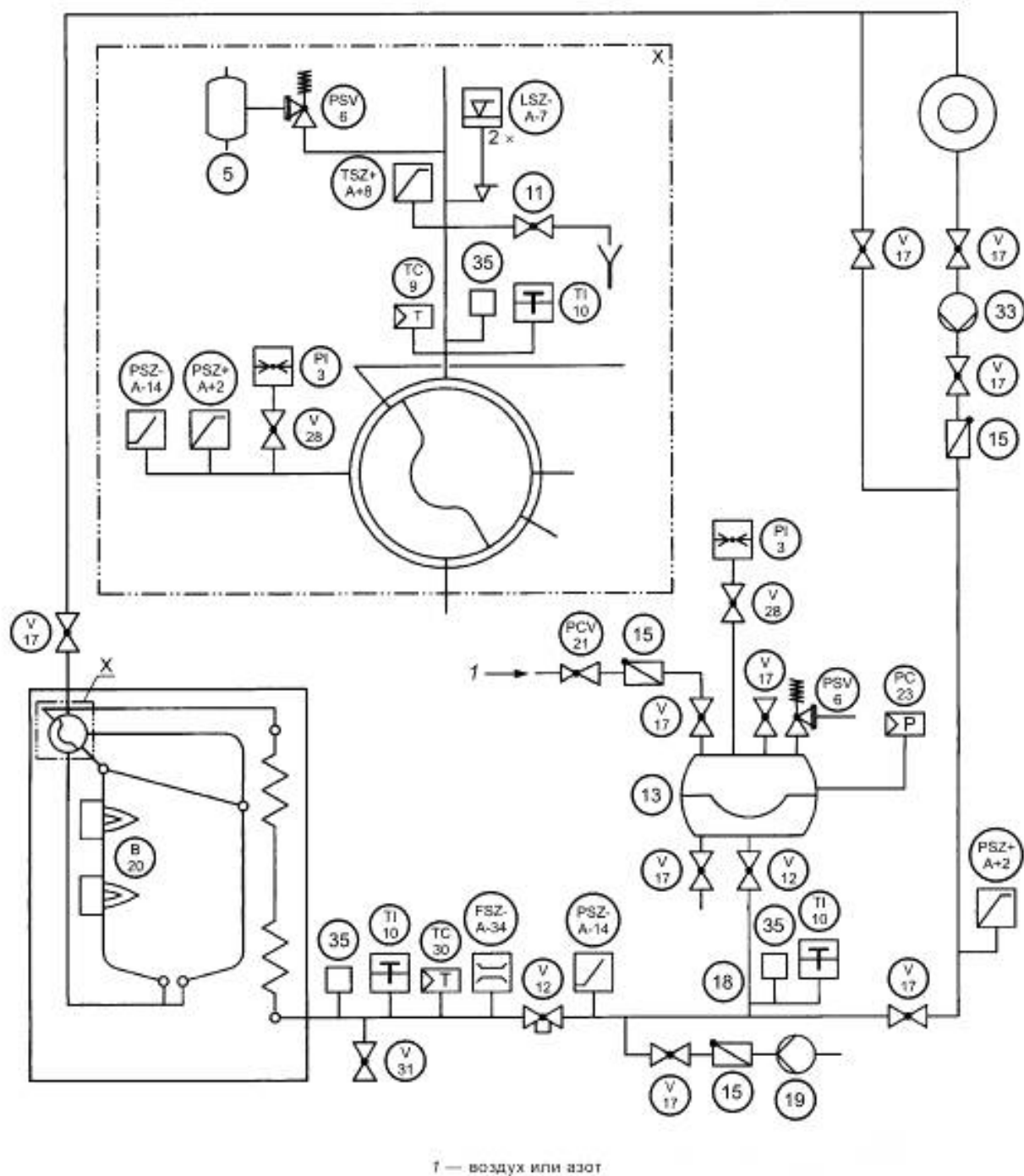
Рисунок В.4-3 — Установки с принудительной циркуляцией, верхней подпиткой воды, поддержанием давления из внешнего источника и газовым аккумулятором
