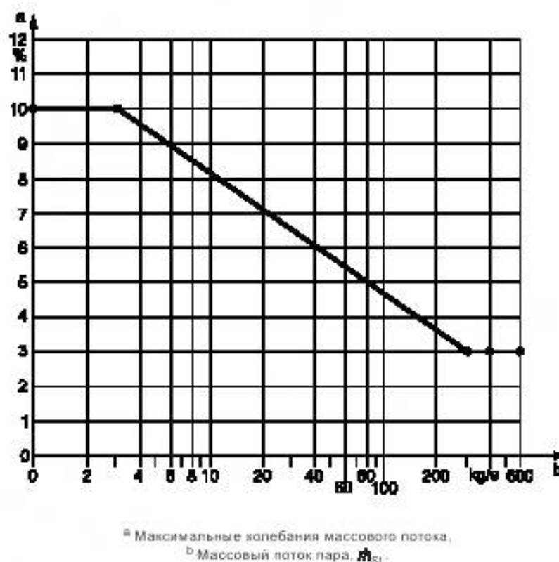
Рисунок 6.6-1 — Максимально допустимые колебания массового потока пара
