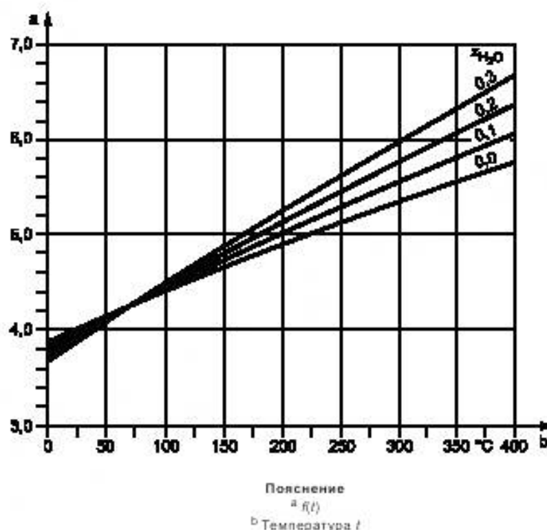
Рисунок 10.4-1 — Функция для расчета коэффициента теплопередачи по линии
