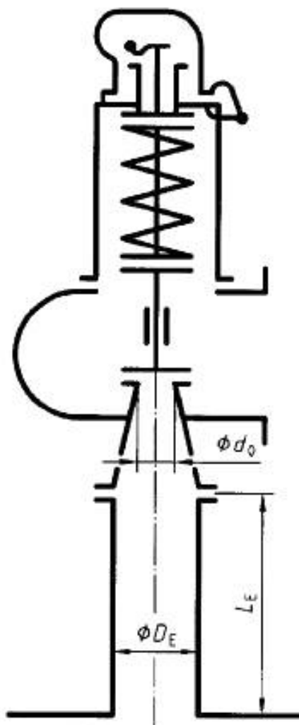
Рисунок 4.1 – Предохранительные клапаны
