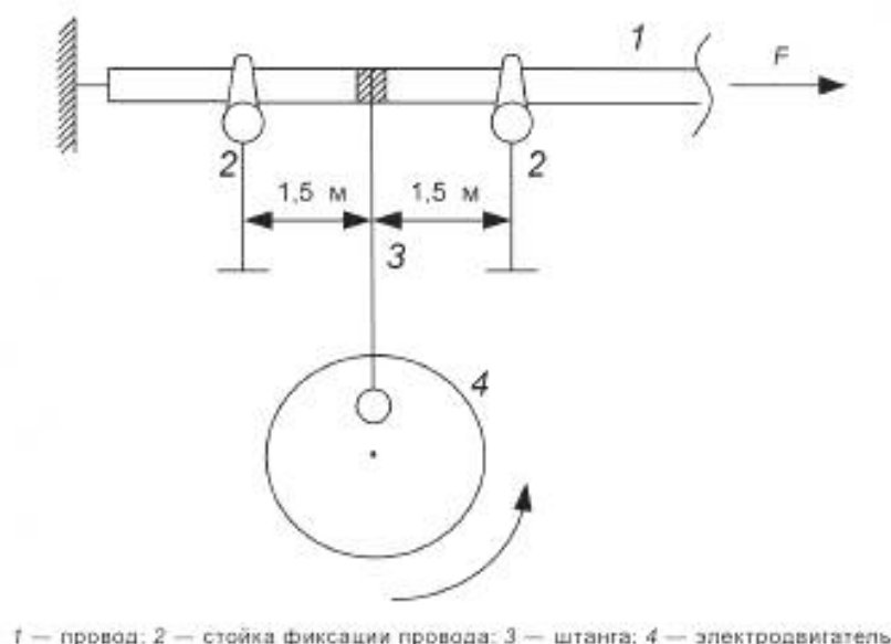
Рисунок 5 — Схема вибрационных испытаний
