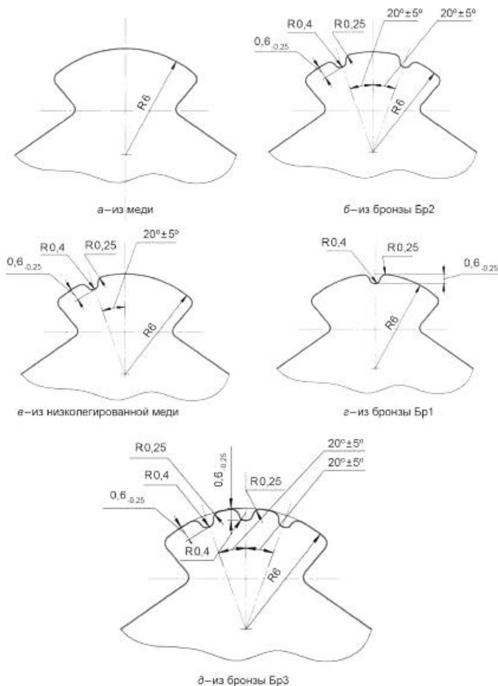
Рисунок 4 — Поперечное сечение провода в зависимости от материала
