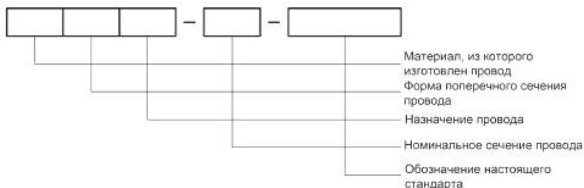
Рисунок 1 — Структурная схема условного обозначения проводов
