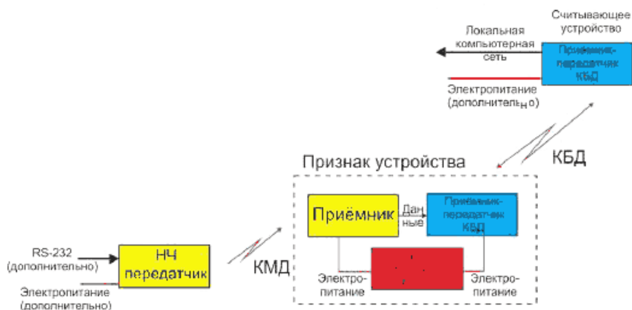
Рисунок 1 – Компоненты системы и их взаимодействие
