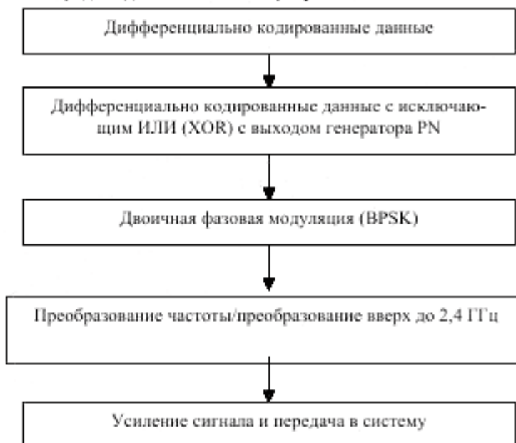
Рисунок 6 – Процесс кодирования и передачи данных передатчика
