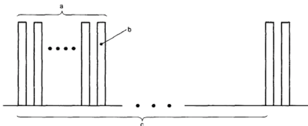
Рисунок 7 – Радиоинтерфейс DSSS
