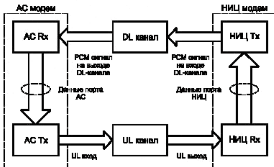
Рисунок В.1 — Общая схема функционирования тональных модемов
