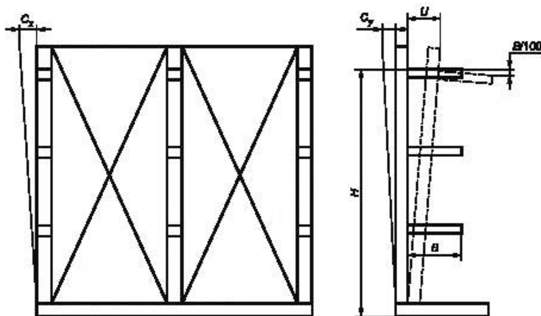
Рисунок 14 — Прогиб элементов консольных стеллажей
