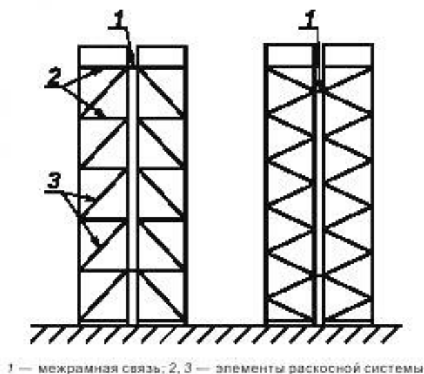
Рисунок 17 — Схема установки межрамных связей
