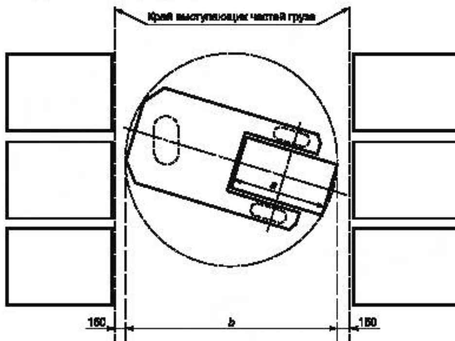
а — длина поддона с грузом; b — габариты ШТ с грузом на захвате
