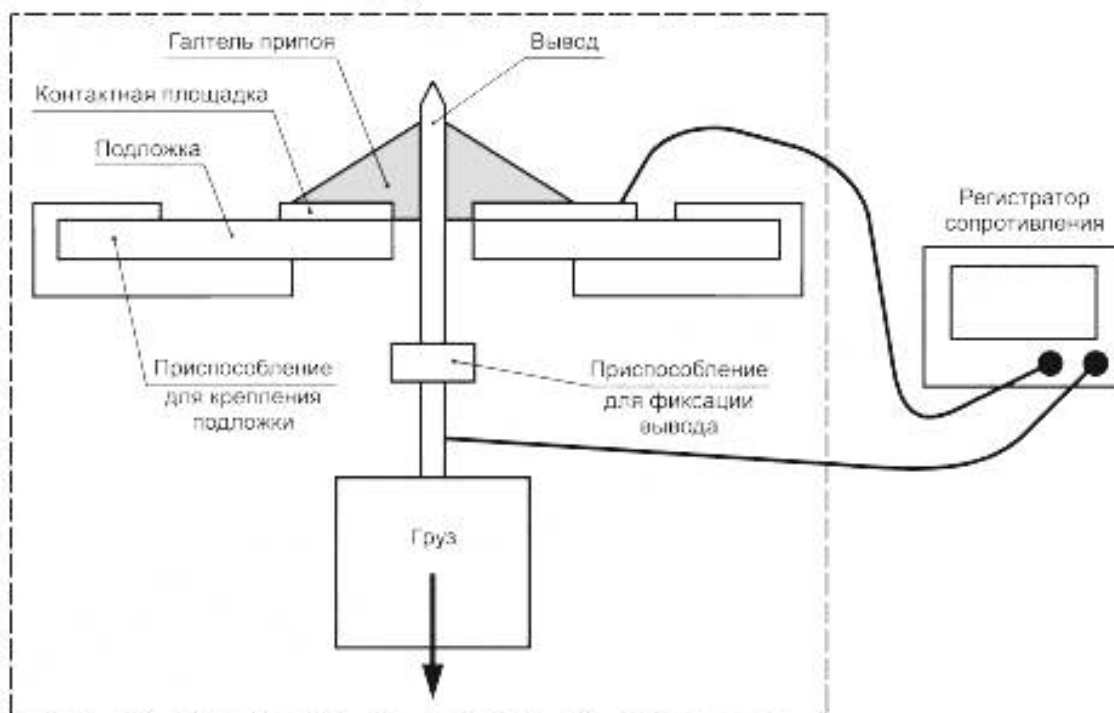
Рисунок G.1 — Испытание на сопротивление ползучести
