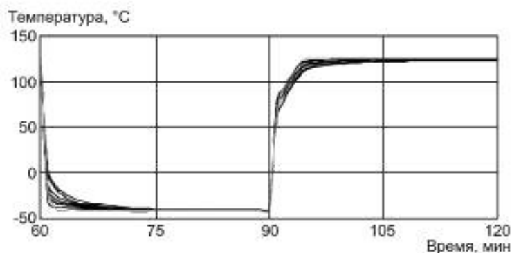
а) Распределение температуры (0 подложек)
