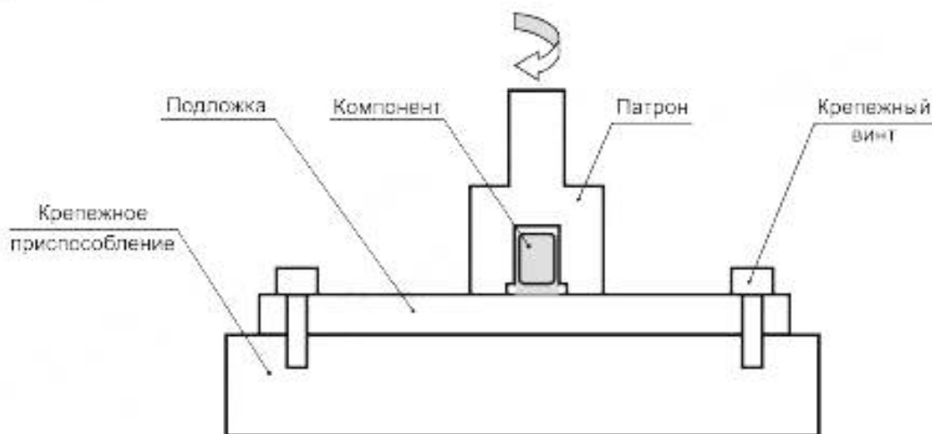
Рисунок 10 — Испытание на прочность при приложении крутящего момента
