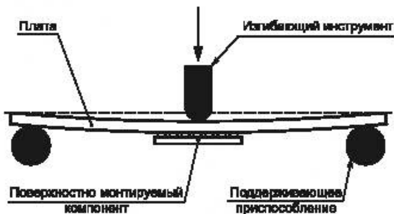
Рисунок D.1 — Пример приспособления для изгиба платы
