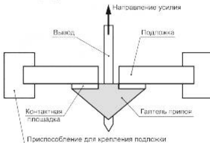
Рисунок F.1 — Испытание прочности на отрыв
