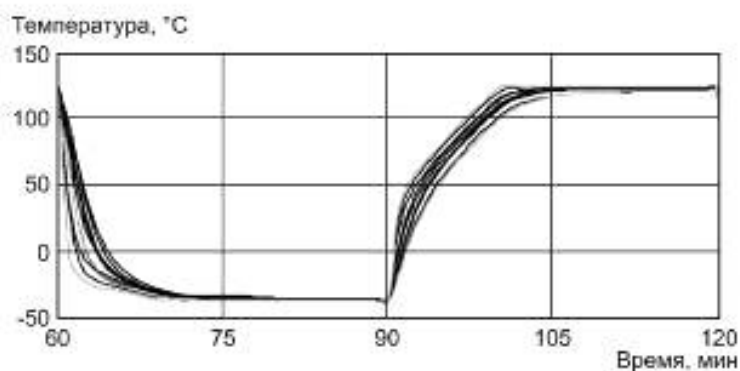
б) Распределение температуры (240 подложек)
