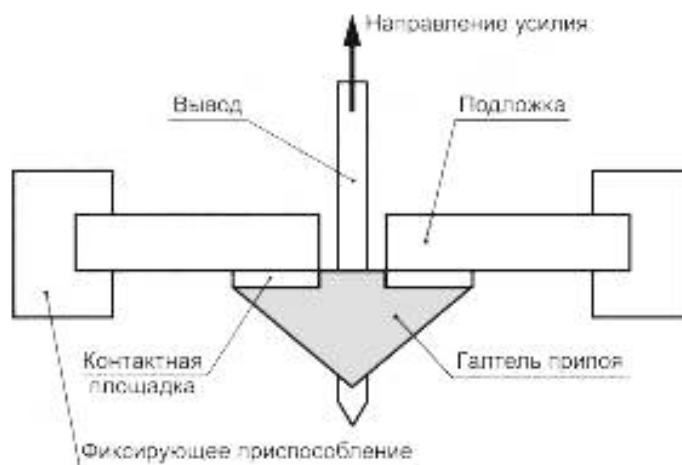
Рисунок 17 — Испытание прочности на отрыв
