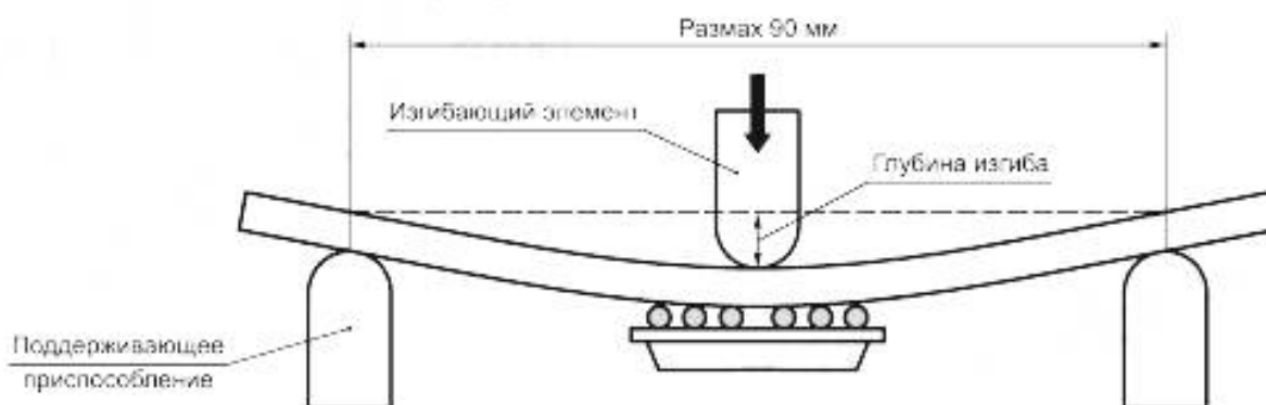
Рисунок 11 — Монотонное испытание на прочность при изгибе
