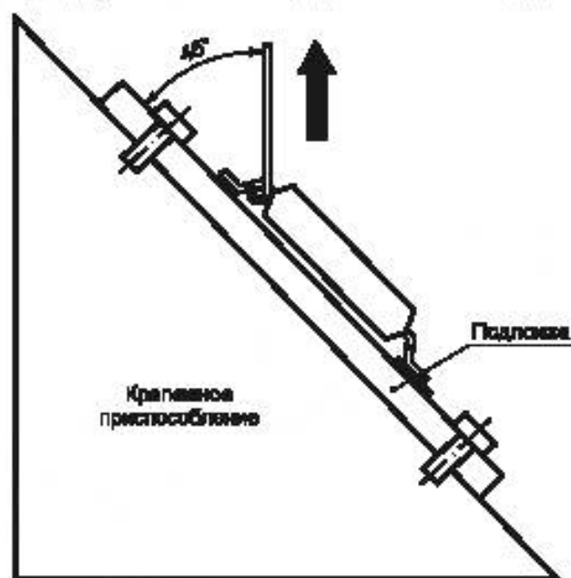
Рисунок 8 — Испытание прочности на отрыв
