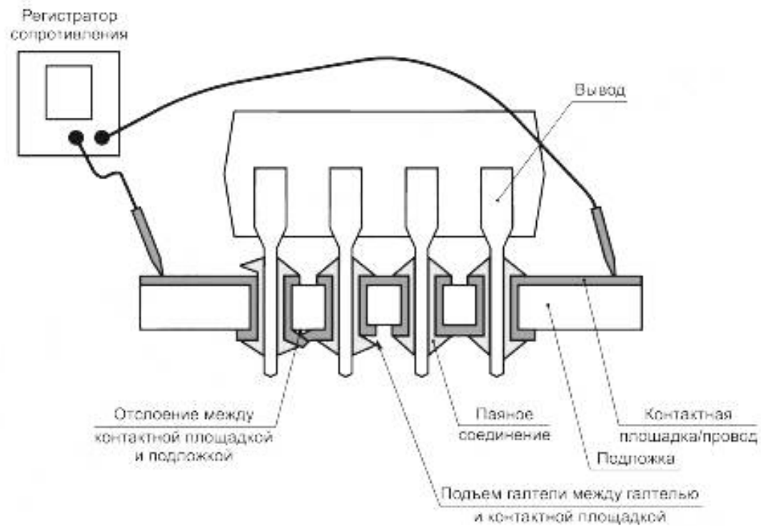
Рисунок Н.2 — Пример схемы для проведения испытаний на наличие электрического соединения в месте пайки для устройства с выводами, монтируемыми в отверстия
