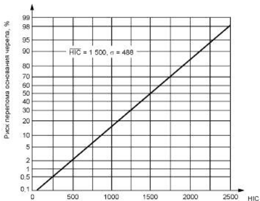
Рисунок А.1 — Риск перелома основания черепа для AIS \geq 2 , как функция HIC при длительности удара 15 мс
