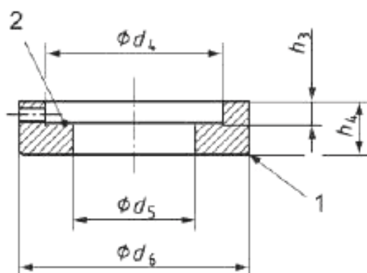
Рисунок А.2 – Промежуточное кольцо, тип А
