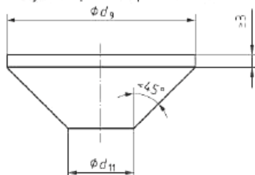
Рисунок А.4 – Нагрузочные опоры
