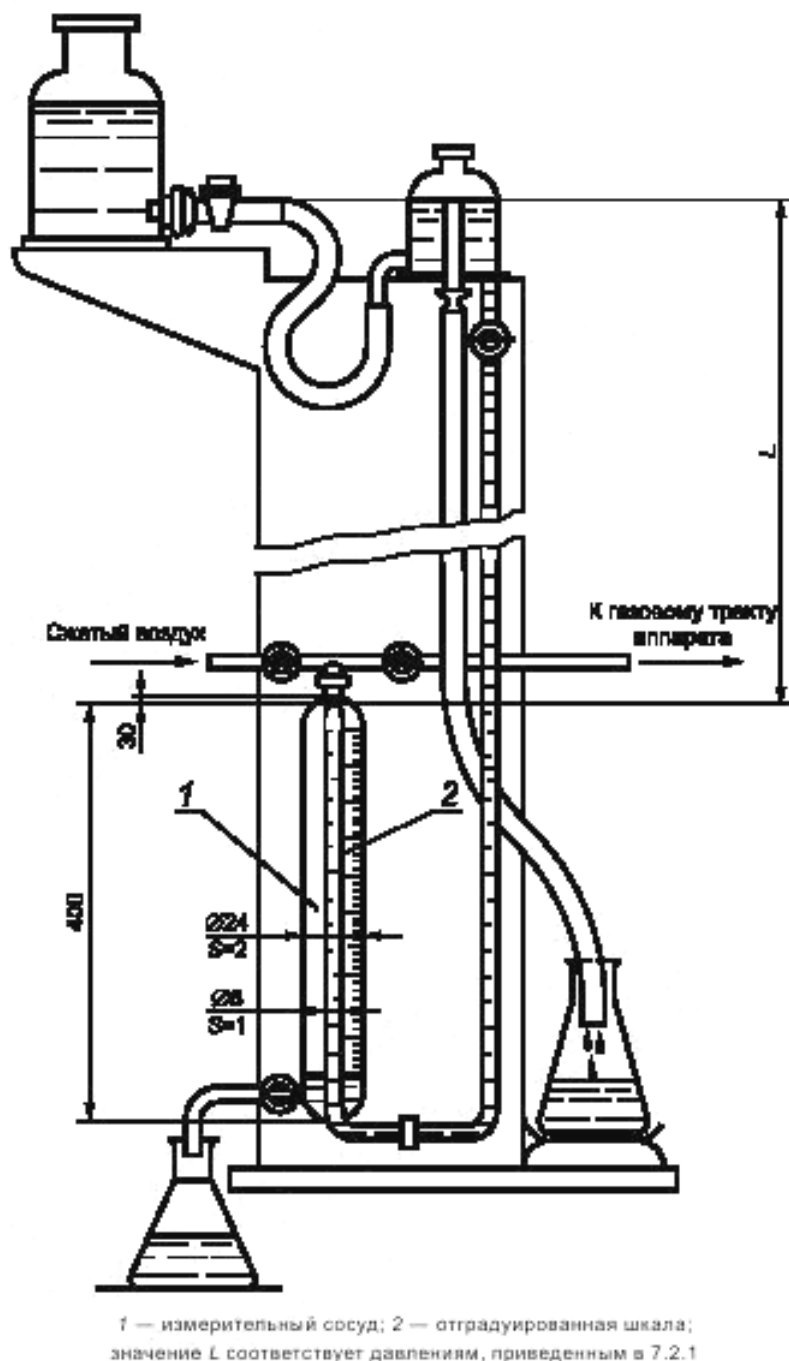
Рисунок 1 — Устройство для проверки герметичности газового тракта
