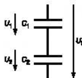
U_0 — напряжение, приложенное к изоляции; U_1 — напряжение, приложенное к изоляционному промежутку; U_2 — напряжение, приложенное к твердой изоляции; C_1 — емкость изоляционного промежутка; C_2 — емкость твердой изоляции
