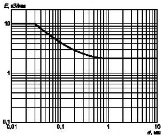
Рисунок 4 — Допустимая напряженность электрического поля для назначения твердой изоляции в соответствии с равенством (7)
