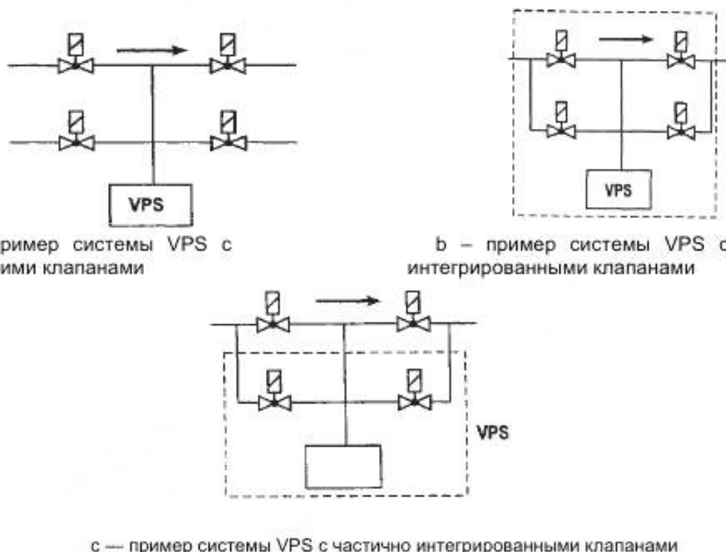
Рисунок 2 — Примеры систем VPS
