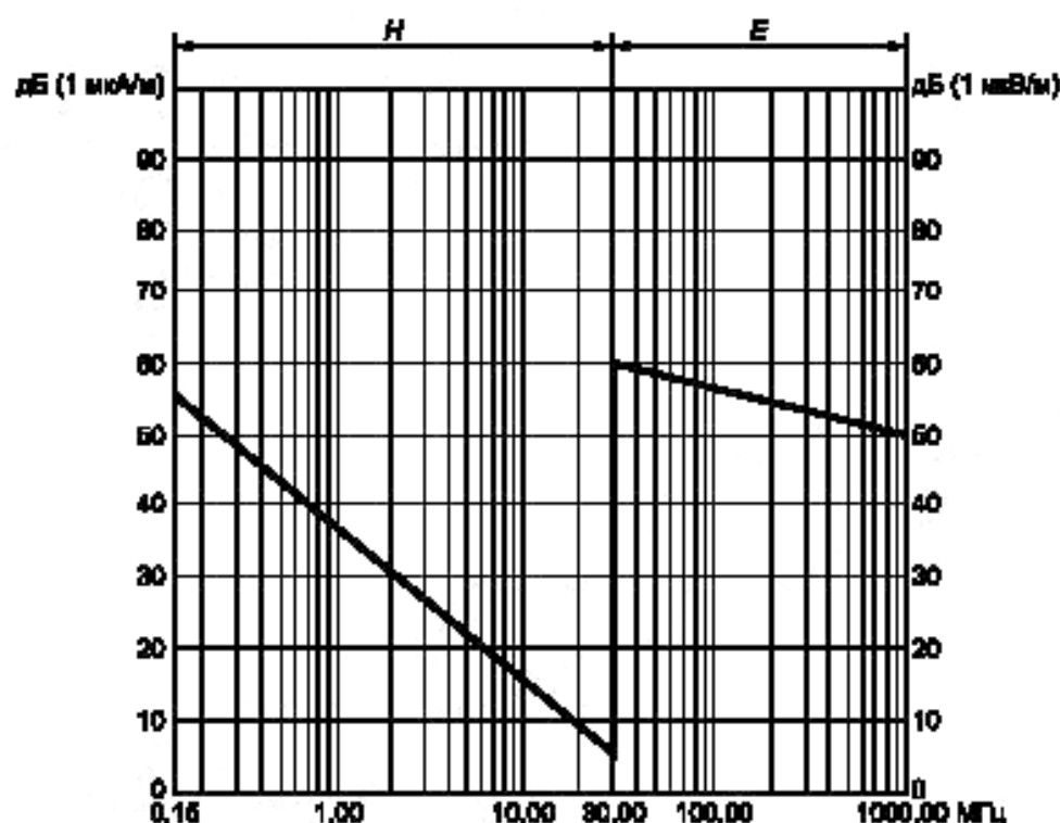
Рисунок 2 — Нормы напряженности поля электромагнитных помех (квaziпиковые значения) от тяговых подстанций
