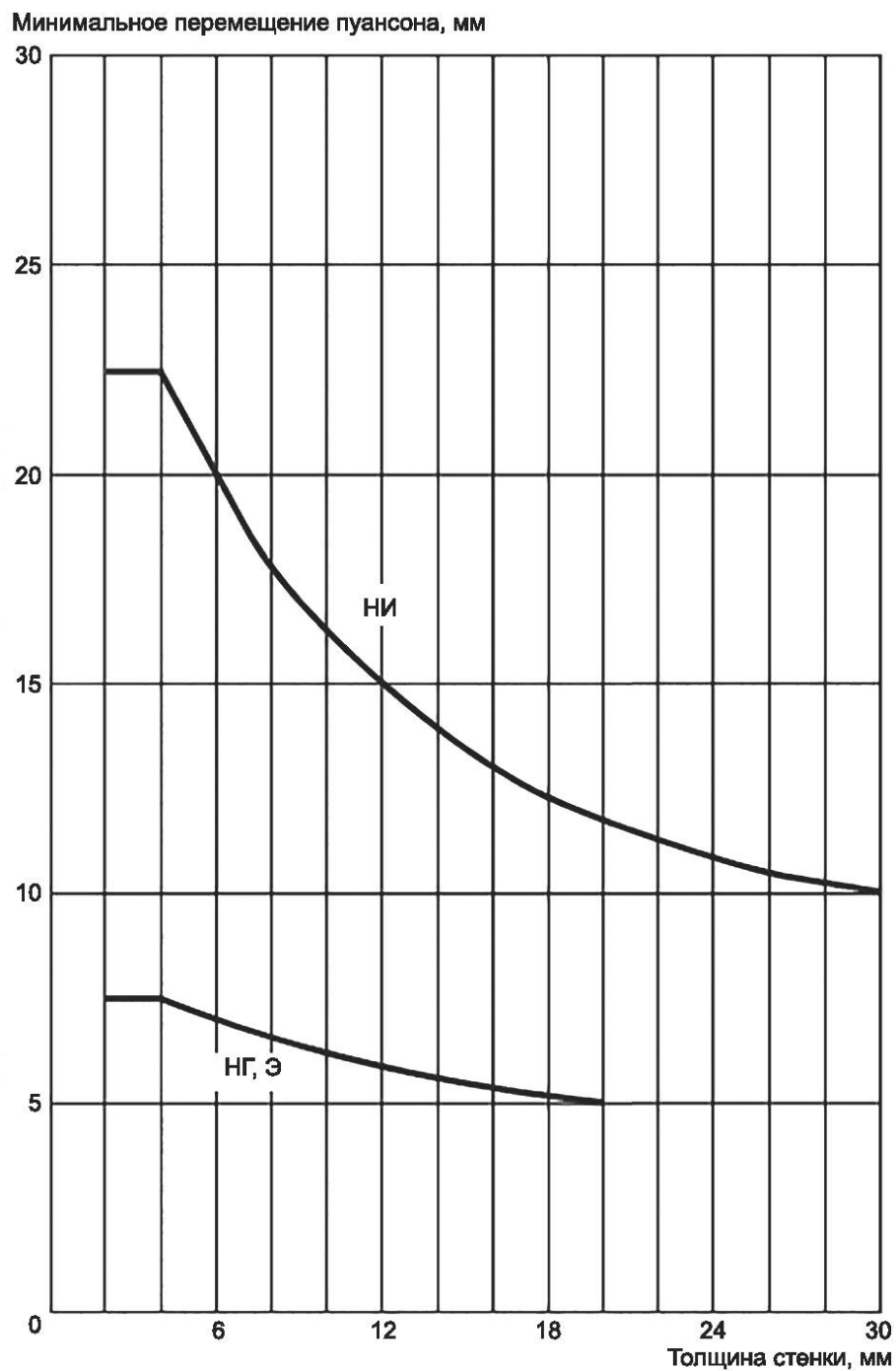
Рисунок Б.11 — Минимальное перемещение пуансона для НПВХ в зависимости от толщины для разных методов сварки (верхняя кривая — для сварки НИ, нижняя — для сварки НГ и Э)
