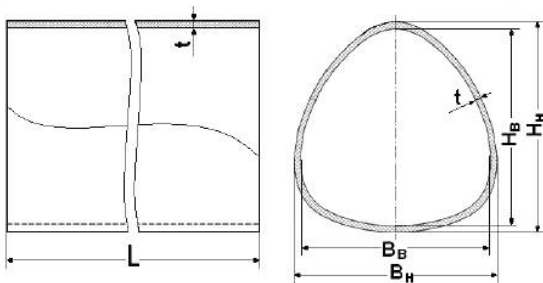
Рисунок 4.1 – Основные размеры сегментов трубопроводов типа К
