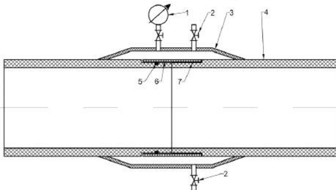
1 – манометр; 2 – вентили впуска/выпуска; 3 – кожух из стеклокомпозита; 4 – сборный узел трубопровода; 5 – уплотнительное кольцо; 6 – муфта; 7 – клеевой состав
