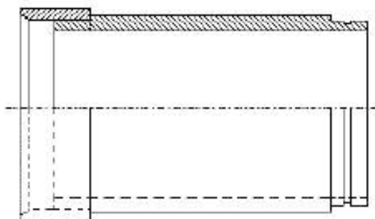
Рисунок 5.1 – Вариант поставки с одной установленной муфтой
