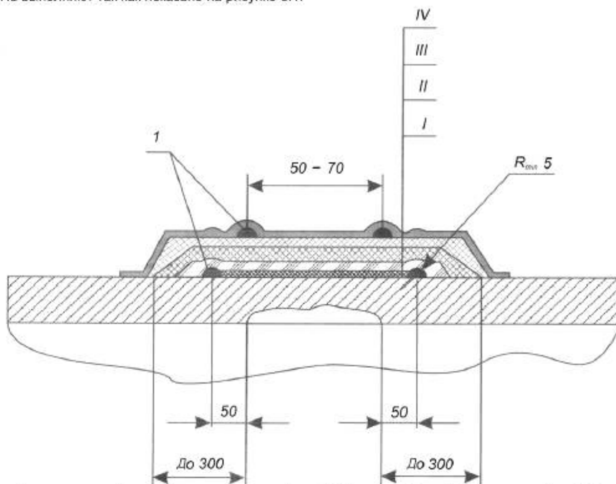
I – специальный слой; II – технологический слой; III – силовой слой; IV – защитный слой; 1 – ровинг; R_{\text{ровн}} – жгут ровинга радиусом не менее 5 мм
