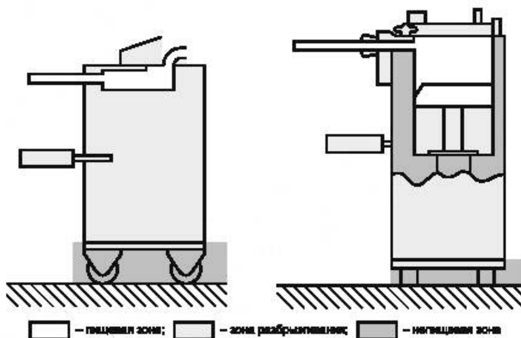
Рисунок 29 — Гигиенические зоны вспомогательных механизмов
