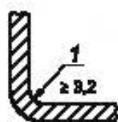
1 — радиус, образованный механической обработкой фасонным резцом
