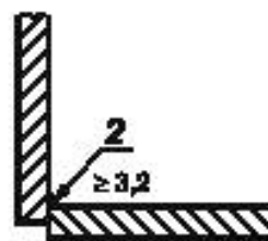
2 — радиус, образованный сварным швом
