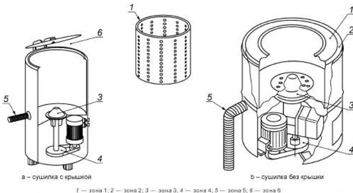
Рисунок 2 — Опасные зоны сушилки
