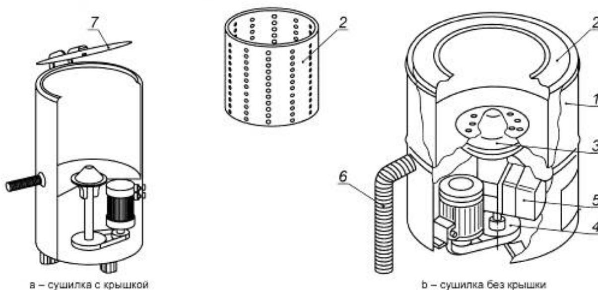
Рисунок 1 — Примеры сушилок
