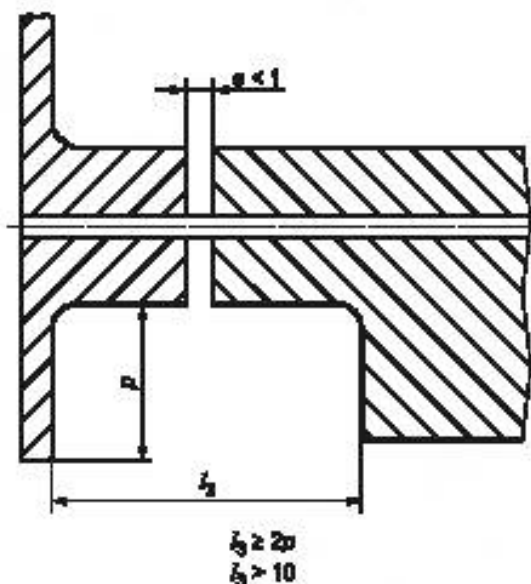
Рисунок А.24 — Шарнирное соединение
