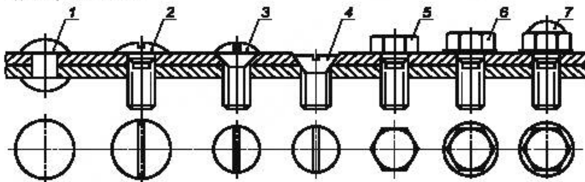
1 – заклепка с полукруглой головкой; 2 – винт с полукруглой головкой; 3 – винт с полукруглой головкой с шлицем; 4 – винт с полукруглой головкой с шлицем; 5 – болт с шестигранной головкой; 6 – болт с шестигранной головкой с коническим подголовком; 7 – винт с шестигранной выпуклой головкой
