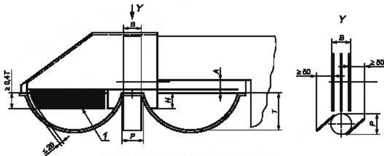
Рисунок 6 – Примеры конструкции куттеров
