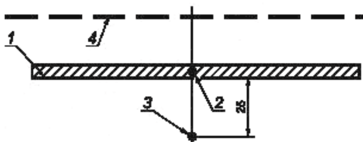
1 — акустический экран; 2 — опорная точка; 3 — контрольная точка в середине акустического экрана; 4 — железнодорожный путь
