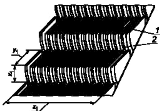
Рисунок 5 — Ступени (основные размеры)
