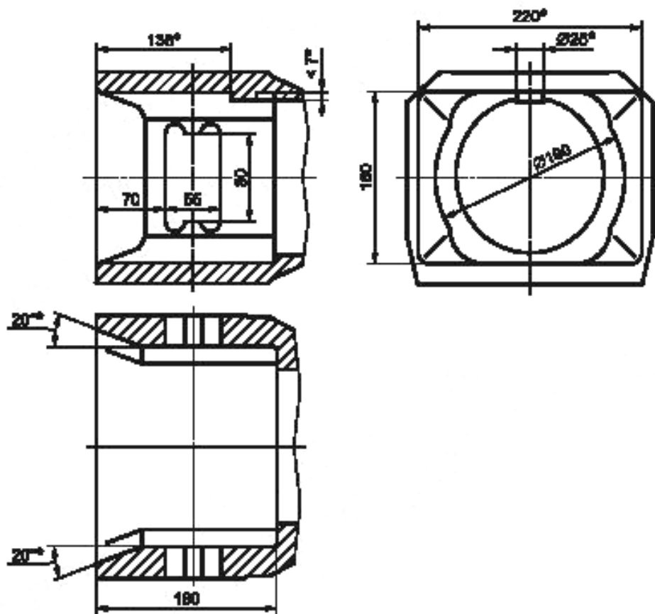
Рисунок А.1 — Корпус сцепки
