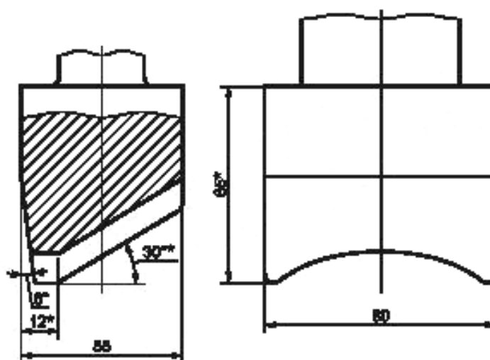
Рисунок А.2 — Замок
