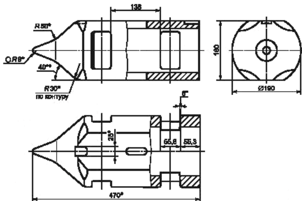
Рисунок А.3 — Направляющий элемент
