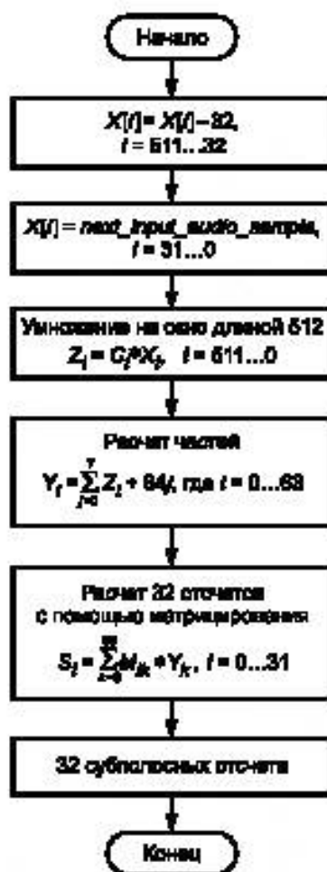
Рисунок В.4 — Блок-схема алгоритма субполосной фильтрации
