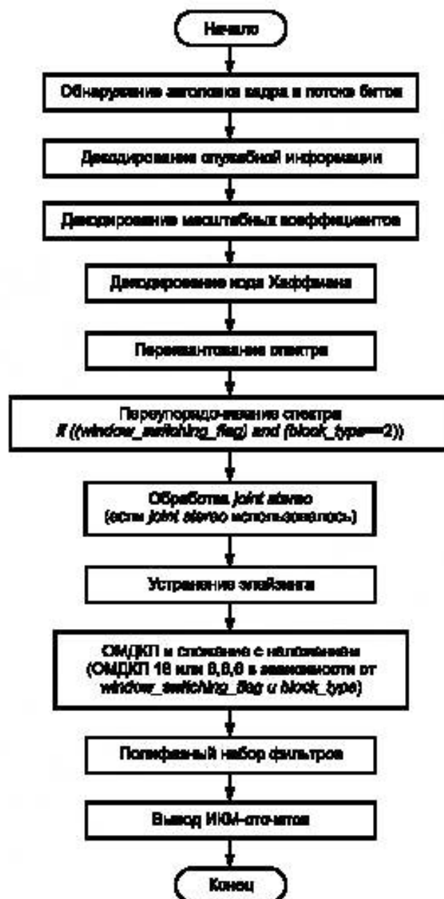
Рисунок А.3 — Блок-схема алгоритма декодера. Уровень III
