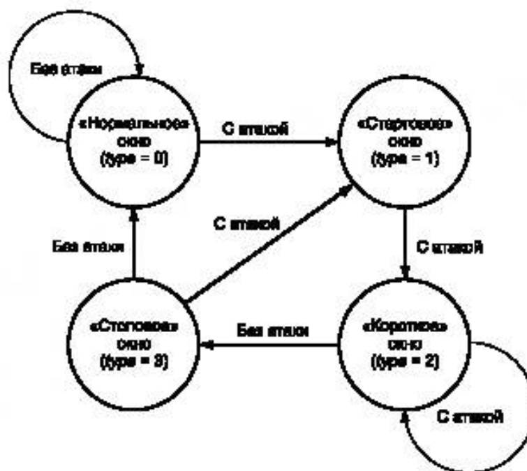
Рисунок В.7 — Граф переключения окон
