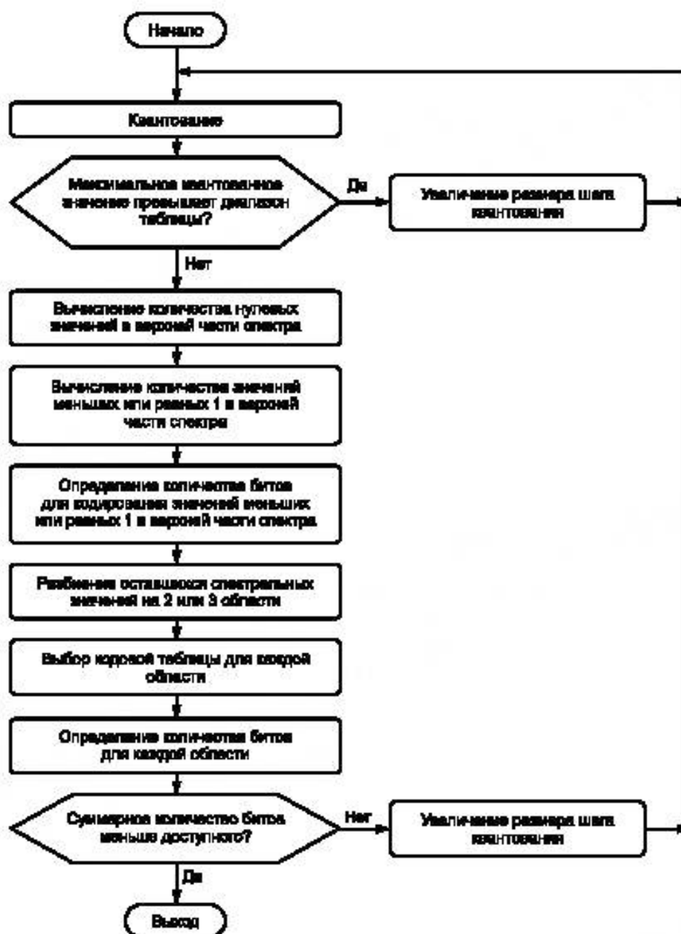
Рисунок В.9в –Внутренний цикл итерации. Уровень III
