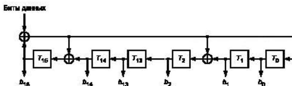
Рисунок А.9 — Схема проверки CRC
