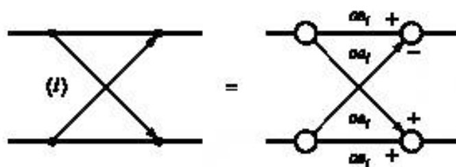
Рисунок А.6 — «Бабочка» устранения злызинга в декодере. Уровень III
