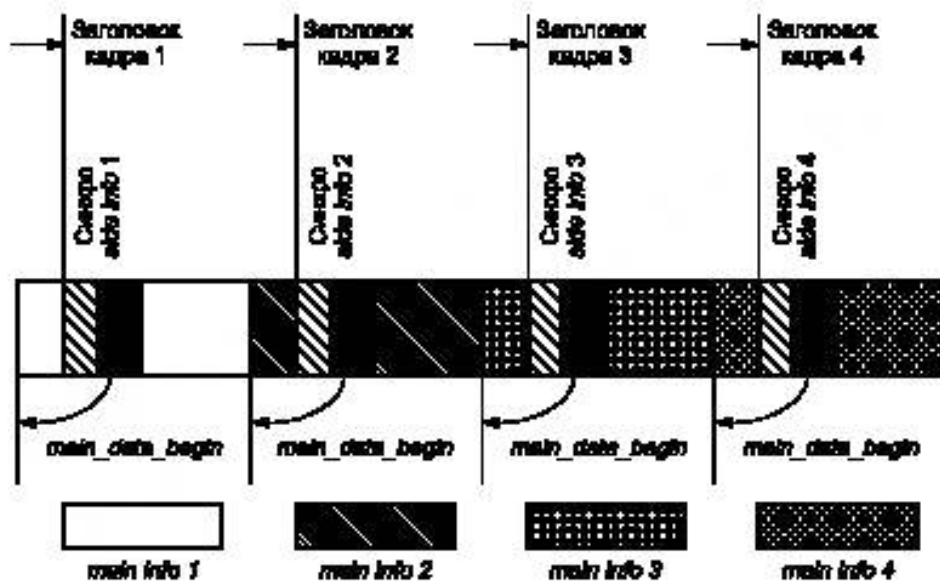
Рисунок А.7.а — Структура потока битов. Уровень III
