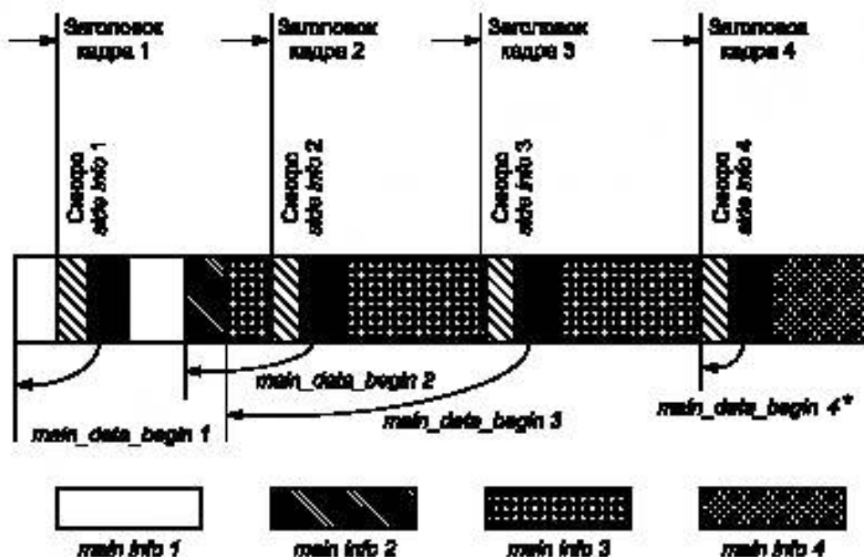
Рисунок А.7.а — Структура потока битов. Уровень III
