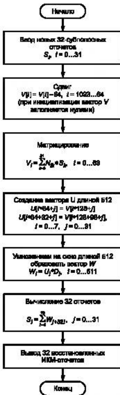
Рисунок А.2 — Блок-схема алгоритма субполосной фильтрации
