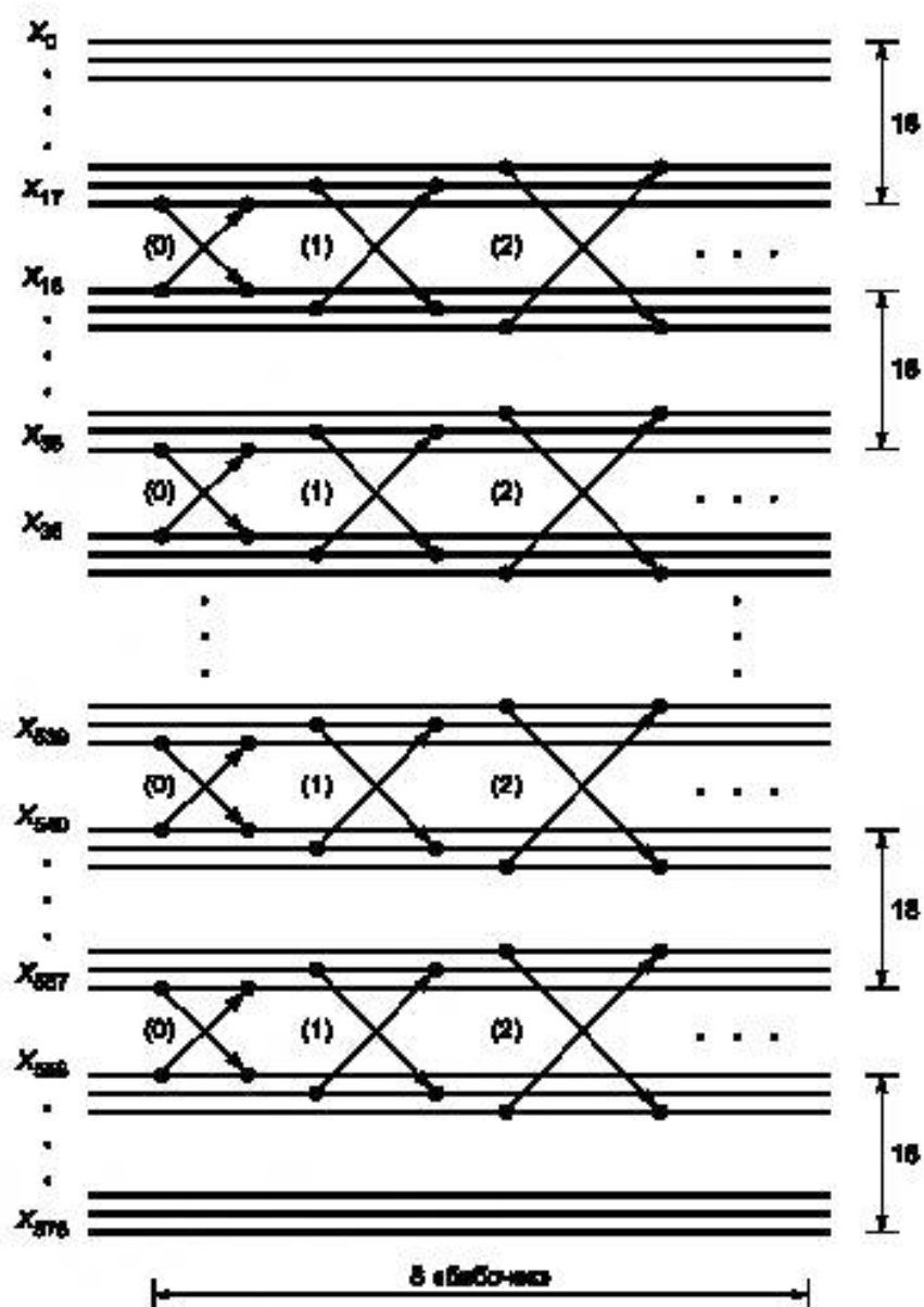
Рисунок А.5 — Диаграмма устранения злызинга в декодере. Уровень III
