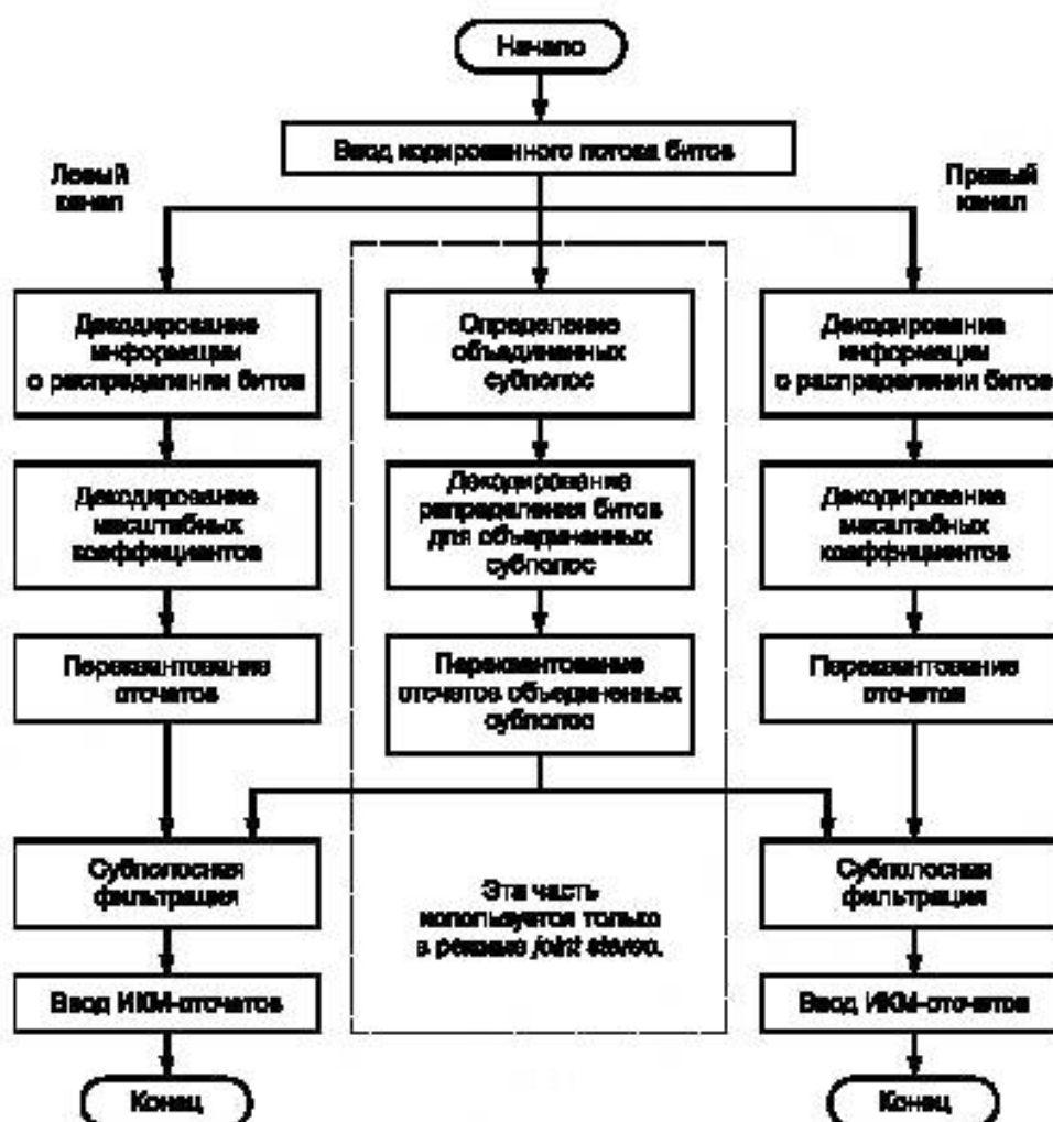
Рисунок Ж.2 — Общая блок-схема декодера стерео
