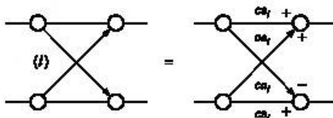
Рисунок В.8 — «Бабочка» в кодере
