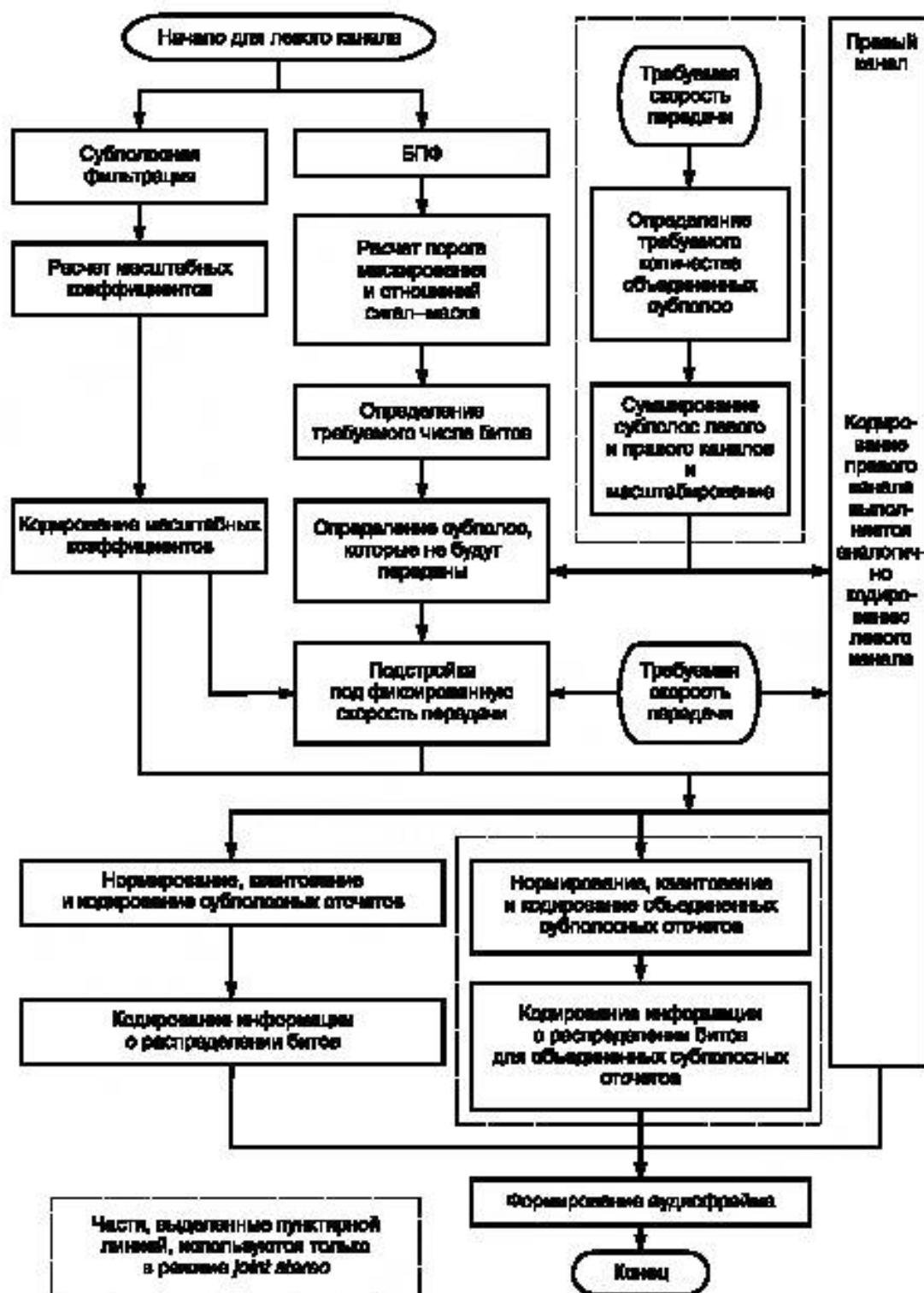
Рисунок Ж.1 — Общая блок-схема кодера стерео
