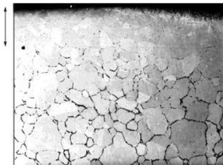
Рисунок 11 — Пример закаленной аустенитной марганцовистой стали, подвергнутой старению при 560^\circ\text{C} в течение 1 ч в целях выделения перлита по границам зерен в тех участках, где содержание углерода выше 1,16\% (номинальное содержание углерода в стали около 1,3\% ) ( 50\times , травление 2 %-ным спиртовым раствором азотной кислоты)
