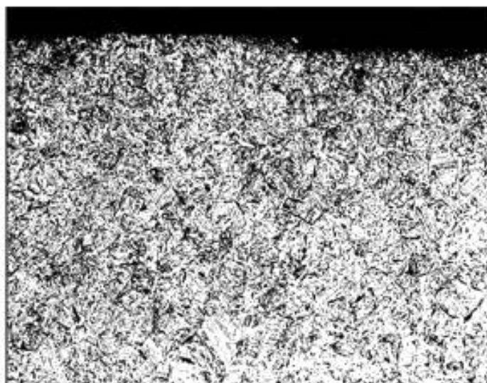
Рисунок 6 — Пример микроstructures (полностью мартенситной) термообработанной легированной стали, в которой не наблюдаются видимые признаки обезуглероживания (200 ×, травление 2 %-ным спиртовым раствором азотной кислоты)
