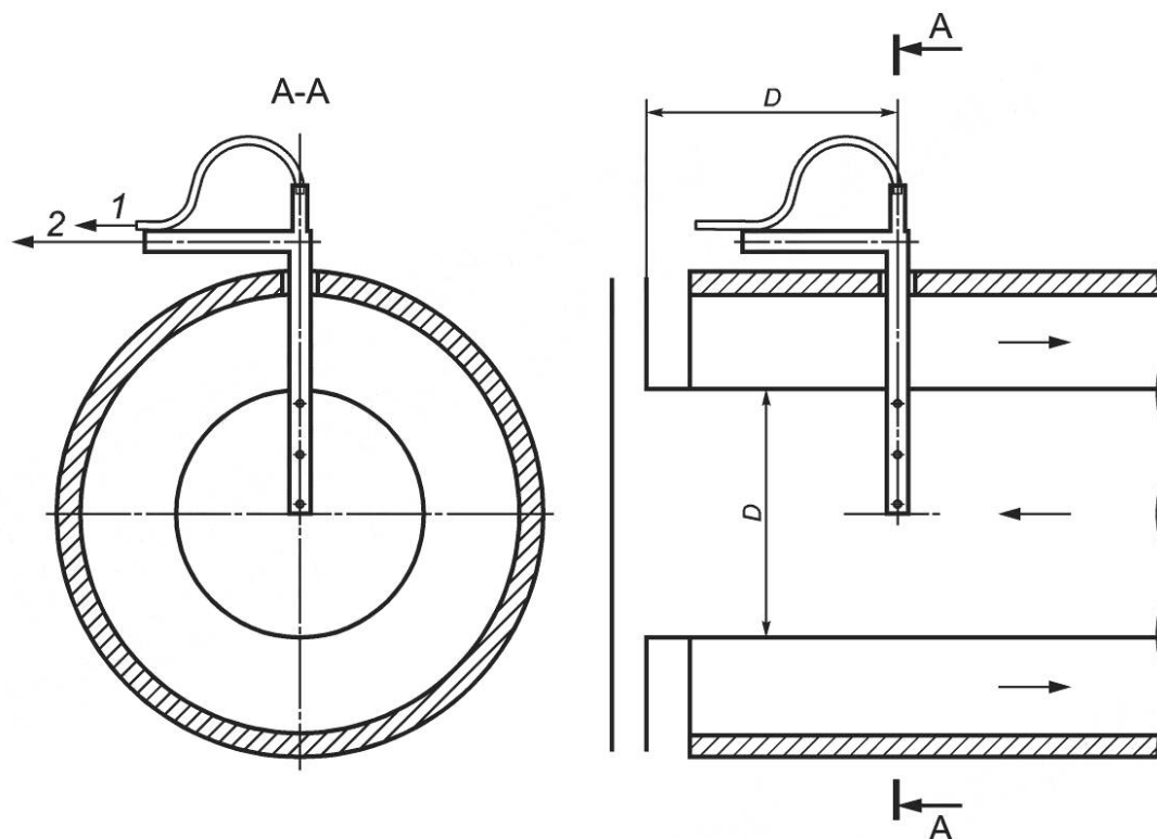
Рисунок М.5 — Расположение испытательного щупа для аппаратов типов C_{12} и C_{13}
