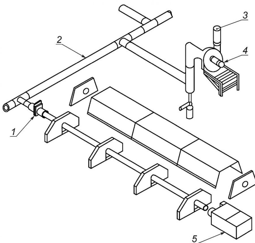
Рисунок В.8 — Системы типа D
