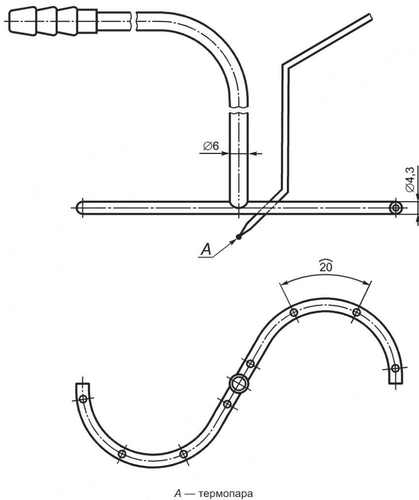
Рисунок М.3 — Пробоотборник для аппаратов типов В 22 , В 23 , В 52 , В 53 , С 32 , С 33 , С 52 и С 53 с диаметром выходного отверстия менее 100 мм
