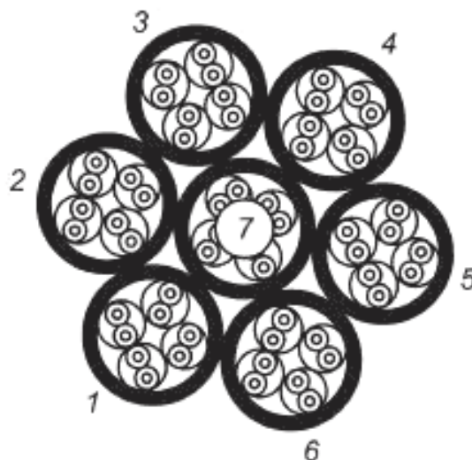
Рисунок 13 — Схема связки из шести кабелей вокруг одного
