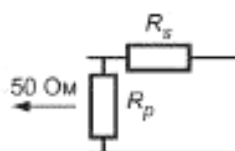
Рисунок 4 — Цепь согласования при Z_k более 50 Ом
