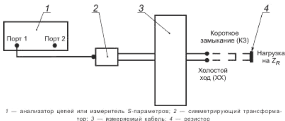
Рисунок 17 — Схема для измерения волнового и входного сопротивлений цепи кабеля и затухания отражения
