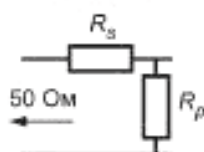
Рисунок 3 — Цепь согласования при Z_k менее 50 Ом
