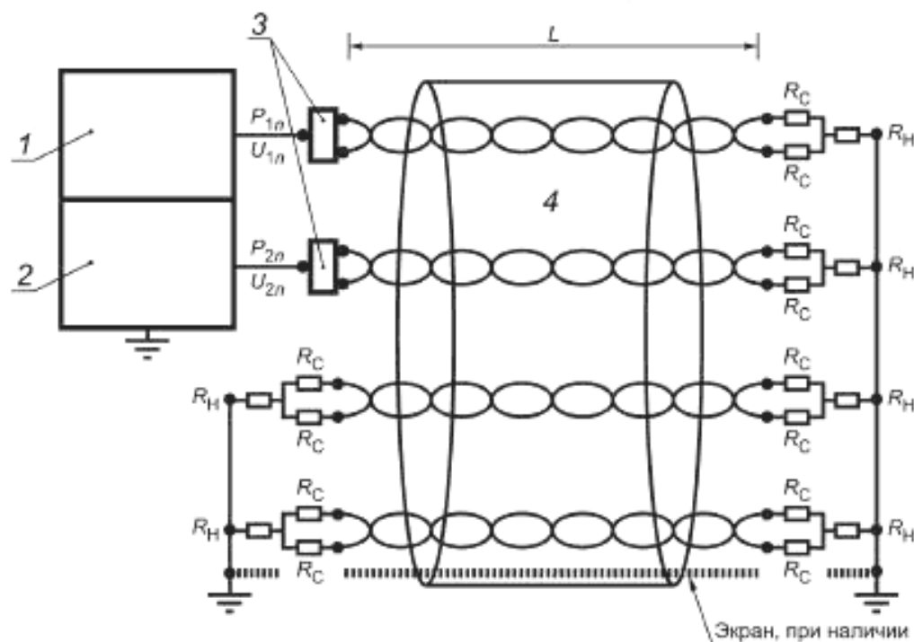
1 — анализатор цепей или генератор сигналов; 2 — анализатор цепей или измерительный приемник; 3 — симметрирующий трансформатор; 4 — измеряемый кабель; R_C и R_N — нагрузки симметричной и несимметричной цепей соответственно; P_{1n}(U_{1n}) — мощность (напряжение) сигнала на ближнем конце влияющей пары; P_{2n}(U_{2n}) — мощность (напряжение) сигнала на ближнем конце подверженной влиянию пары
