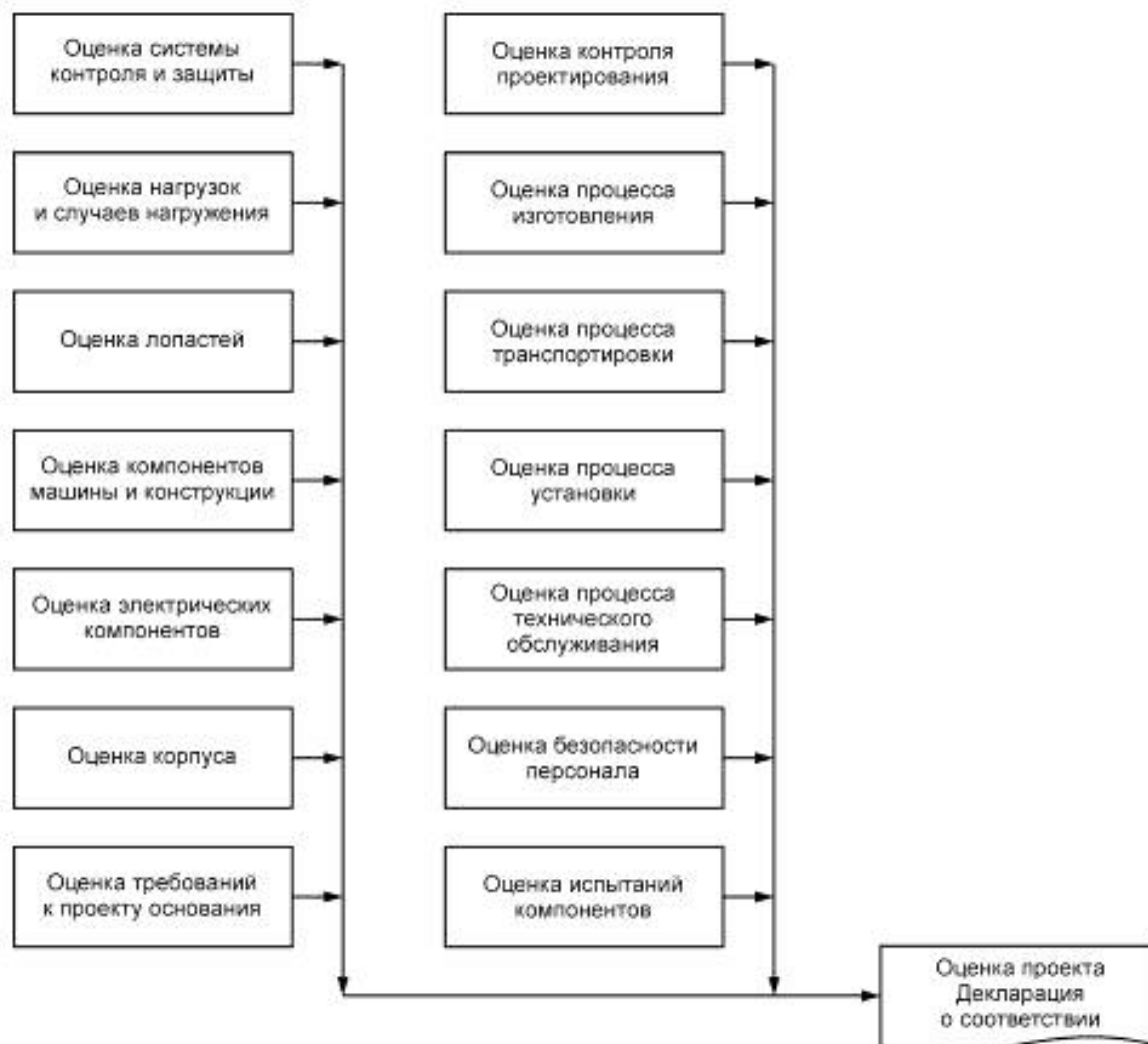
Рисунок 4 — Блок-схема процедуры оценки конструкции ВЗУ
