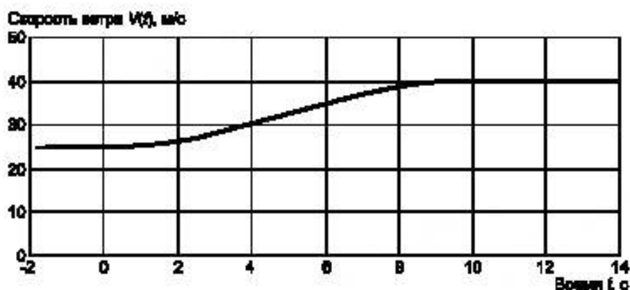
Рисунок 7 — Пример ЭКГ ветра ( V_{hub} = 25 м/с)
