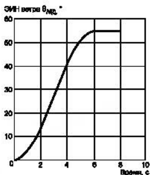
Рисунок 6 — Пример ЭИН ветра ( N = 50 , V_{hub} = 25 м/с)
