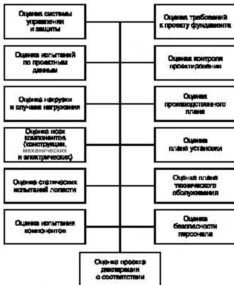
Рисунок А.2 — Элементы оценки проекта
