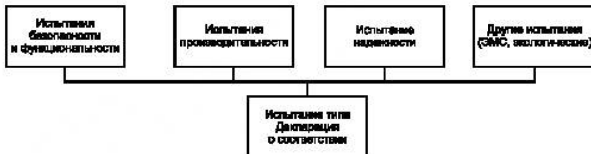
Рисунок А.3 — Элементы испытаний типа
