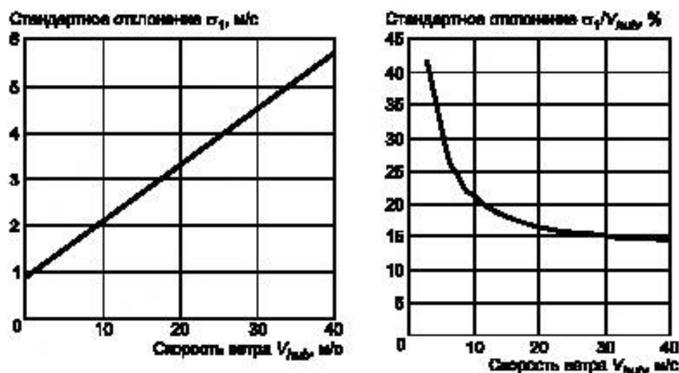
Рисунок 3 — Стандартные отклонения и интенсивность турбулентности в МНТ
