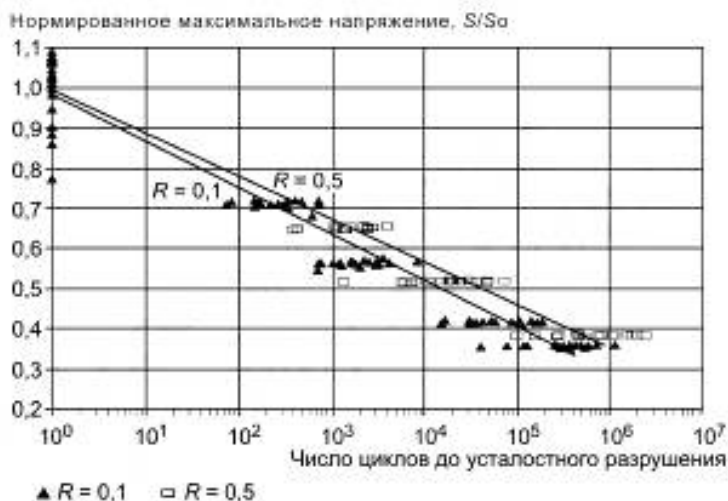
Рисунок Д.2 — Характерные усталостные кривые S - N для композиционного материала на основе стекловолокна
