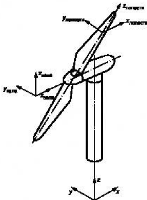
Рисунок 2 — Определение систем координат для компонентов горизонтально-осевой ВЭУ
