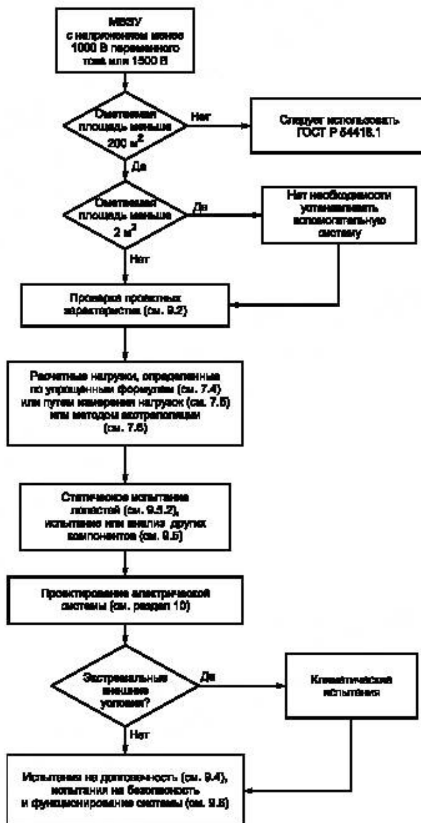
Рисунок 1 — Алгоритм метода проектирования МВЭУ
