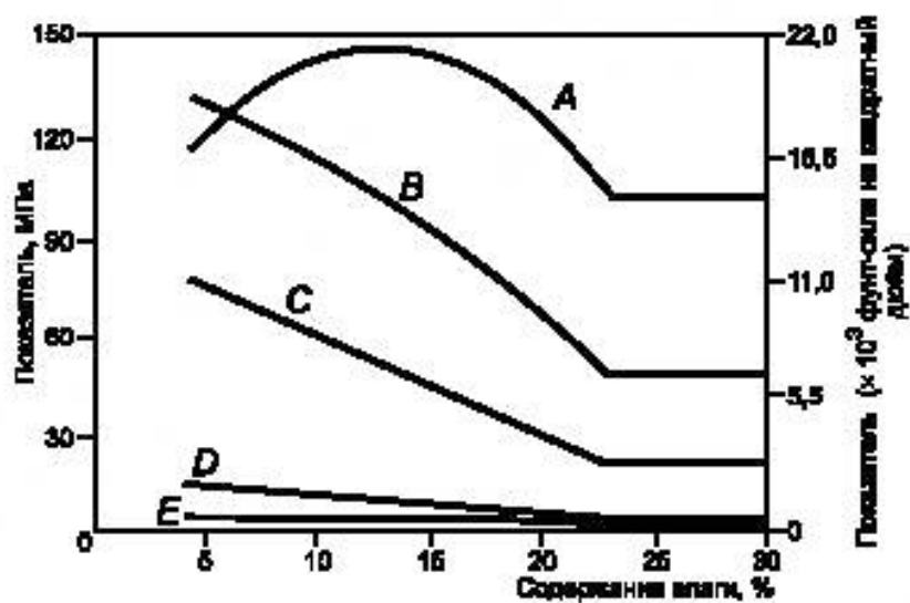
Рисунок Д.8 — Зависимость предельной прочности (при сжатии до образования щепок) древесины от влажности
