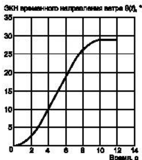
Рисунок 9 — Пример переходного процесса изменения направления ветра ( V_{hub} = 25 м/с)
