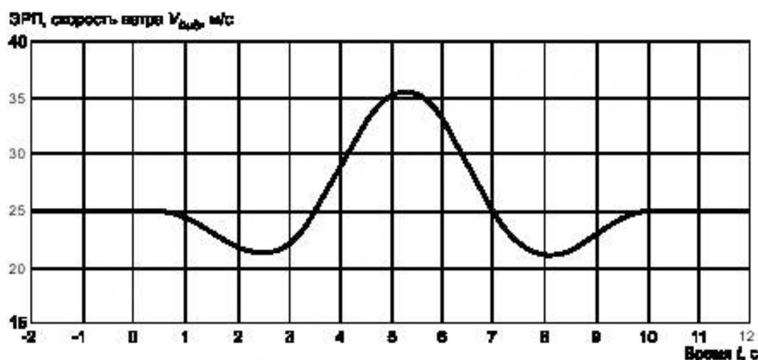
Рисунок 4 — Пример экстремального рабочего порыва ( N = 1 , V_{hub} = 25 м/с)
