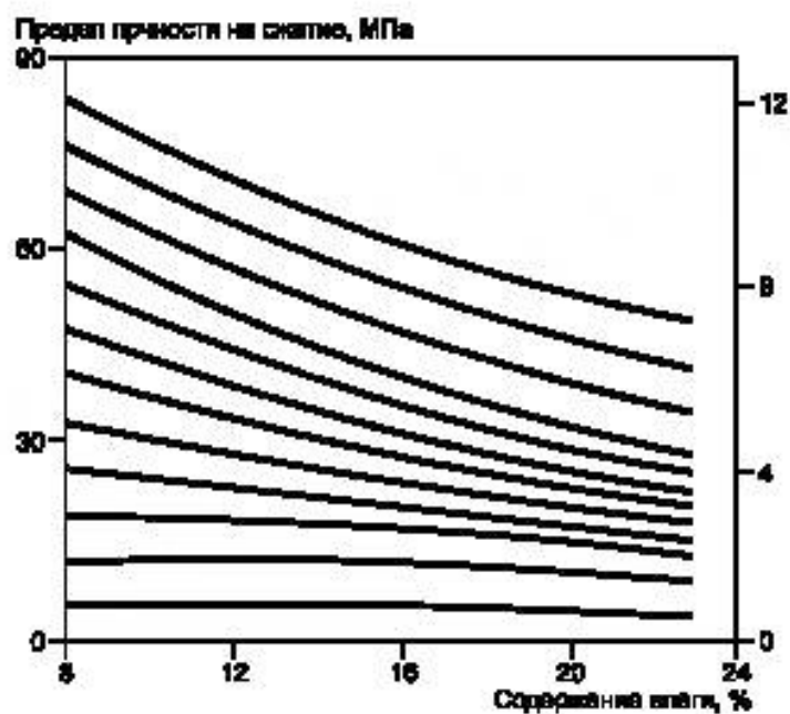
Рисунок Д.8 — Зависимость предельной прочности (при сжатии до образования щепок) древесины от влажности
